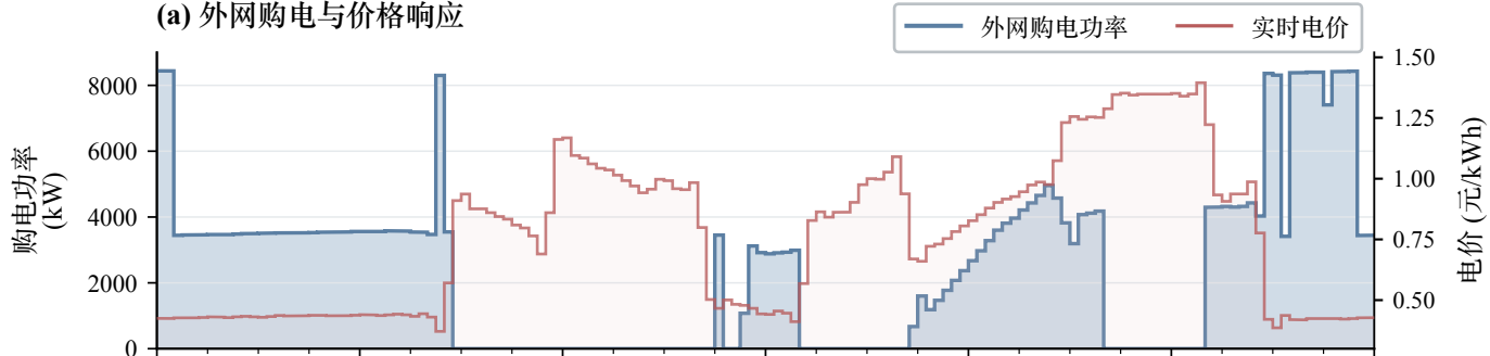
(a) 外网购电与价格响应
