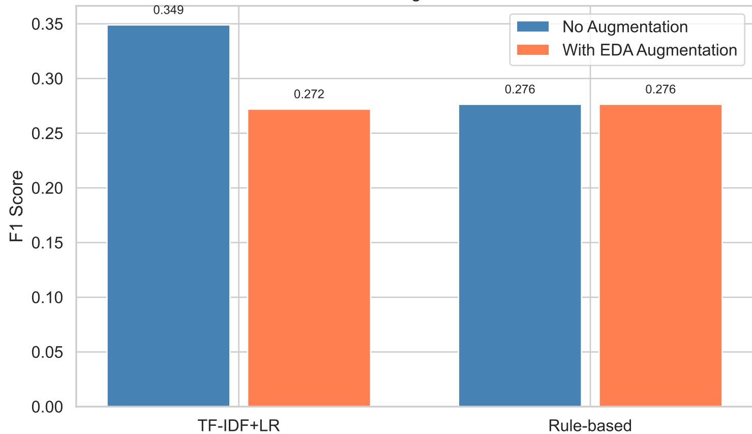
Effect of Data Augmentation on F1
