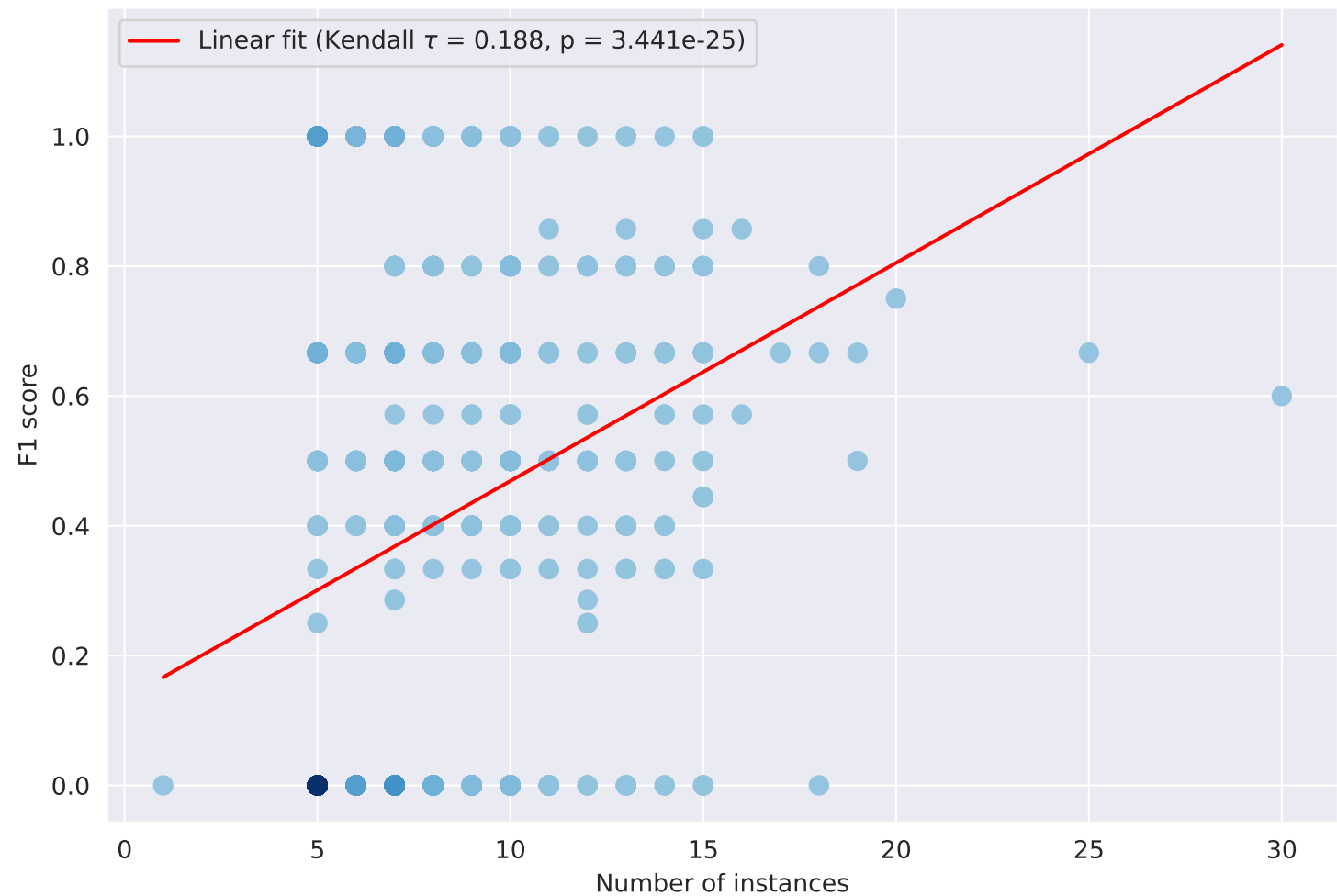
Per-gloss instance count vs. recognition F1 score
