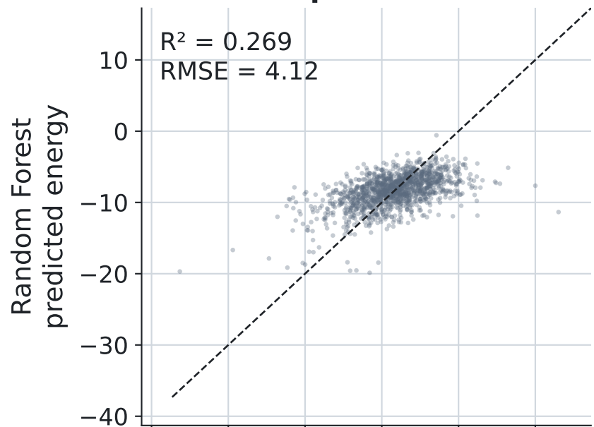
DFT descriptors
