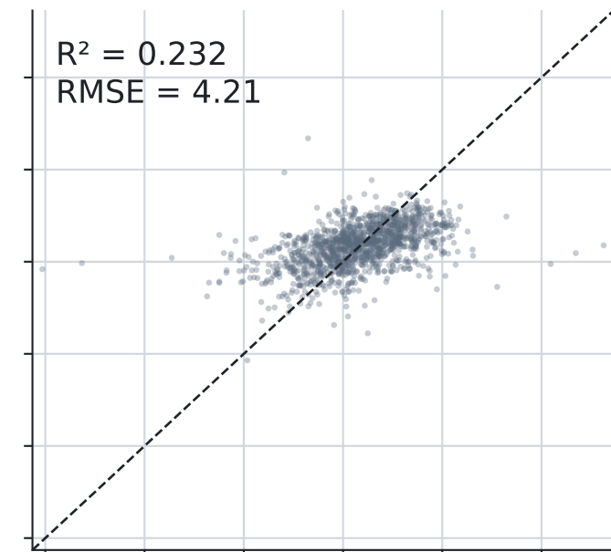
Mordred
