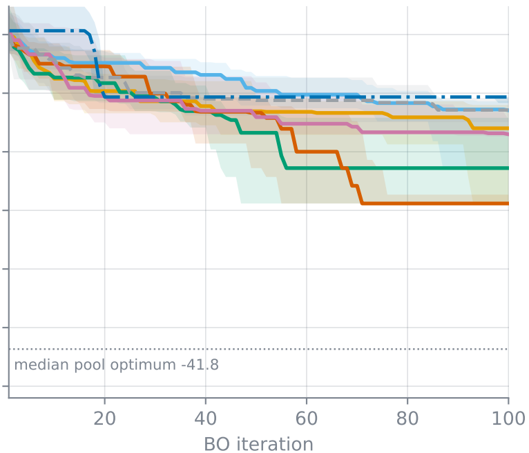
Mordred
