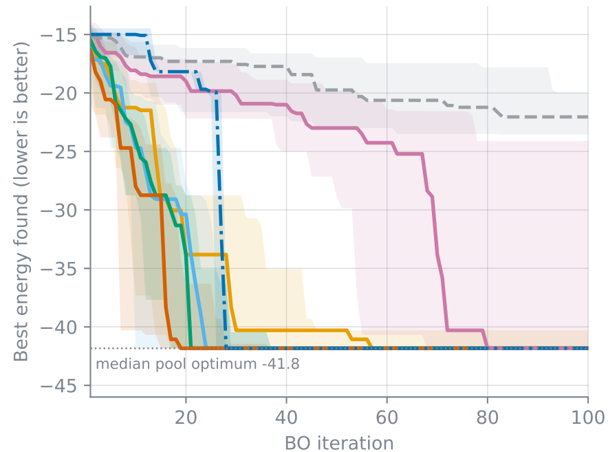
DFT descriptors
