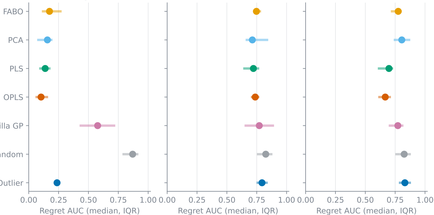
DFT descriptors
