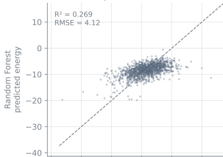
DFT descriptors
