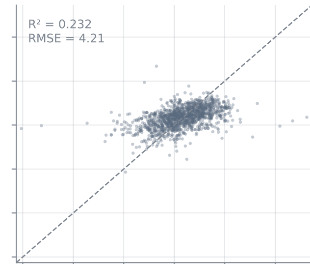
Mordred
