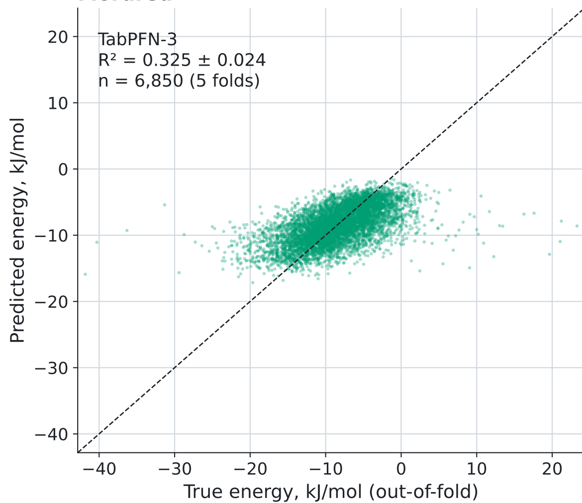
Mordred
