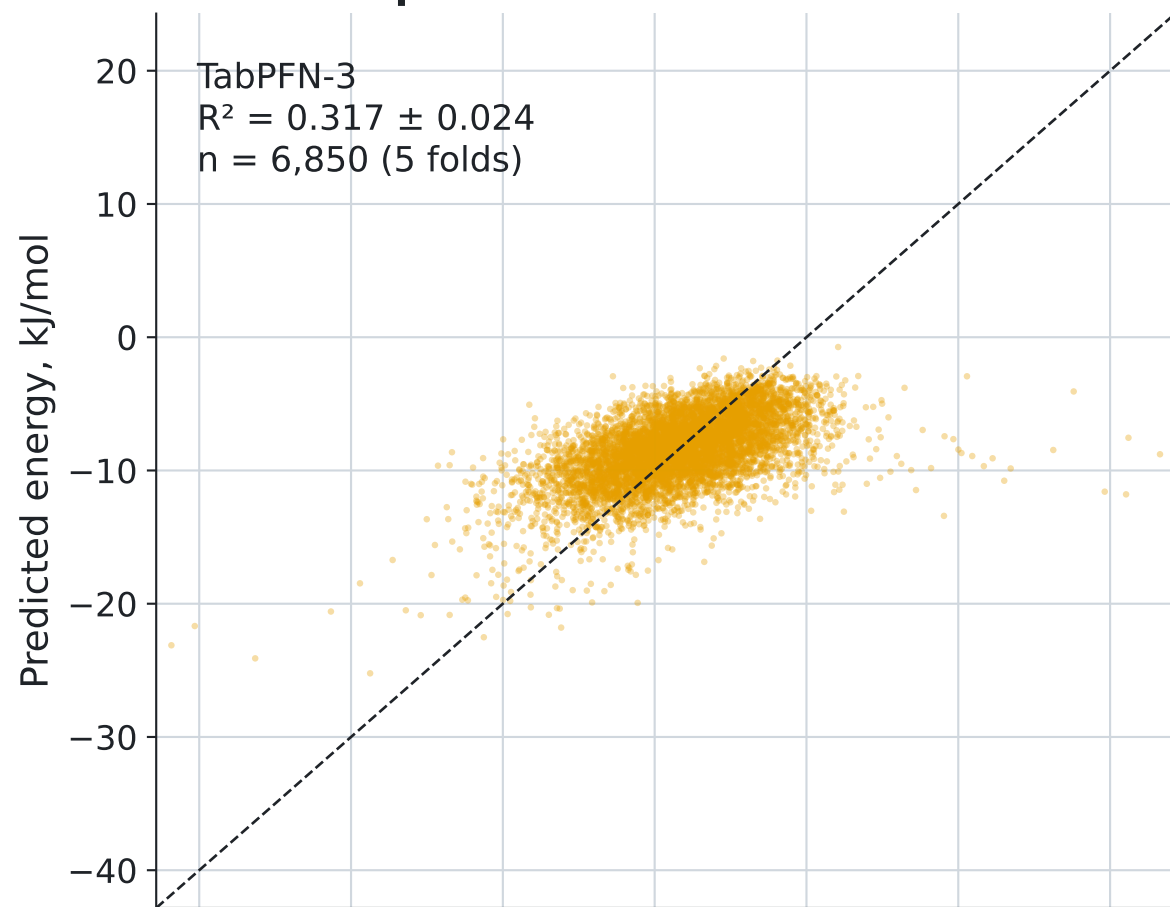
DFT descriptors
