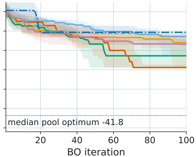
Mordred
