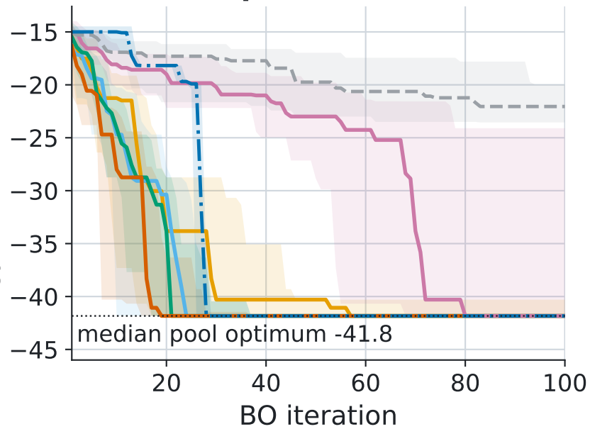
DFT descriptors
