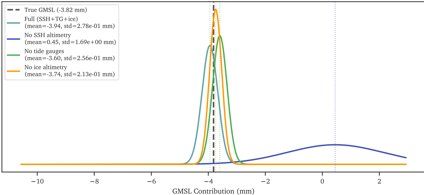
Knockout Test: GMSL Posterior Distributions
