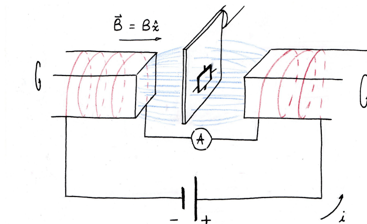
Fig. 1.1: Diagramma in cui viene rappresentato schematicamente l'apparato sperimentale. L'amperometro disegnato misura la corrente che fluisce all'interno delle bobine facendo sviluppare il campo magnetico nel traferro. La sonda di Hall è inserita nel mezzo e ai suoi capi misuriamo tensione V_H e corrente i_p .
