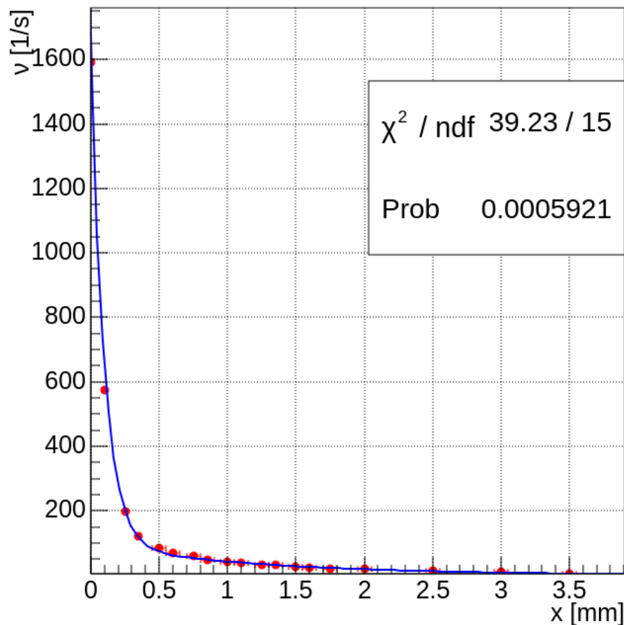
Fig. 3.3: Fit di Lambert-Beer
