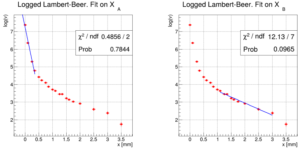
Fig. 3.2: In blu, le regressioni lineari ai logaritmi delle frequenze \log \nu misurate al variare dello spessore di alluminio x (dati in tab. 3.1). A sinistra nella regione X_A = [0, 0.35]\text{mm} e a destra in quella X_B = [1.1, 3]\text{mm} (parametri a cui convergono le regressioni in eq. (3.4) e eq. (3.5)).
