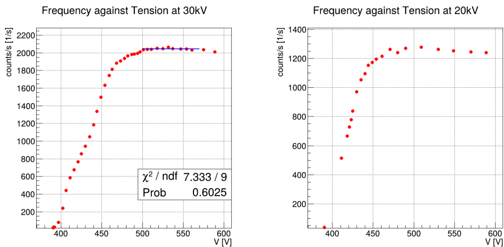
Fig. 2.2: Andamento della frequenza di conteggi (misurata in intervalli di \Delta t = 20s ) al variare della tensione di alimentazione del contatore Geiger (dati in table 2.1). A sinistra i dati relativi a V_{EHT} = 30kV con in blu la curva della regressione sul plateau (modello eq. (2.1), e risultati in legenda), e a destra quelli con V_{EHT} = 20kV .
