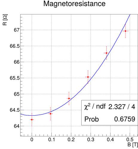
Fig. A.1: Regressione con il modello eq. (A.1) ai dati in tab. A.2: il risultato del fit è in blu. Le resistenze sono espresse in \Omega mentre i valori di campo magnetico sono stati convertiti in T.
