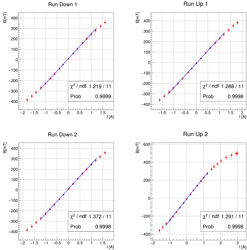
Fig. 2.2: Curve di salita e discesa dei cicli di isteresi (con il campo magnetico B in mT e la corrente nelle bobine I in A): in rosso i dati, e in blu le curve delle regressioni lineari (parametri del fit in legenda). Abbiamo limitato i range dei fit alle regioni di linearità delle curve.
