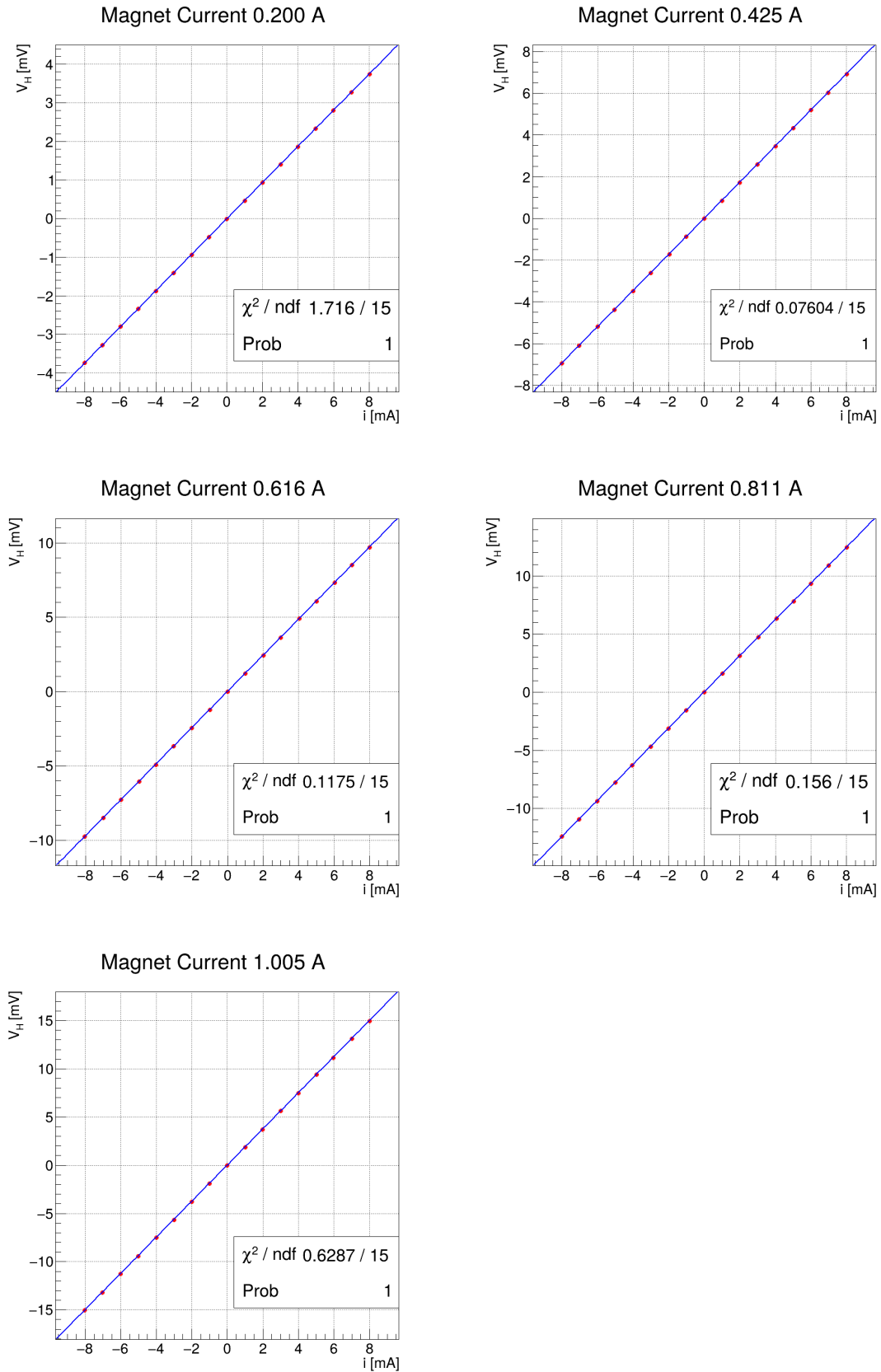
Fig. 3.2: Regressioni (in blu, con parametri dei fit in legenda) all'andamento della tensione di Hall V_H (in mV) contro la corrente nella sonda i_p (in mA) al variare del campo magnetico esterno (determinato dalla “magnet current” nel titolo, indicata più precisamente nel seguito).
