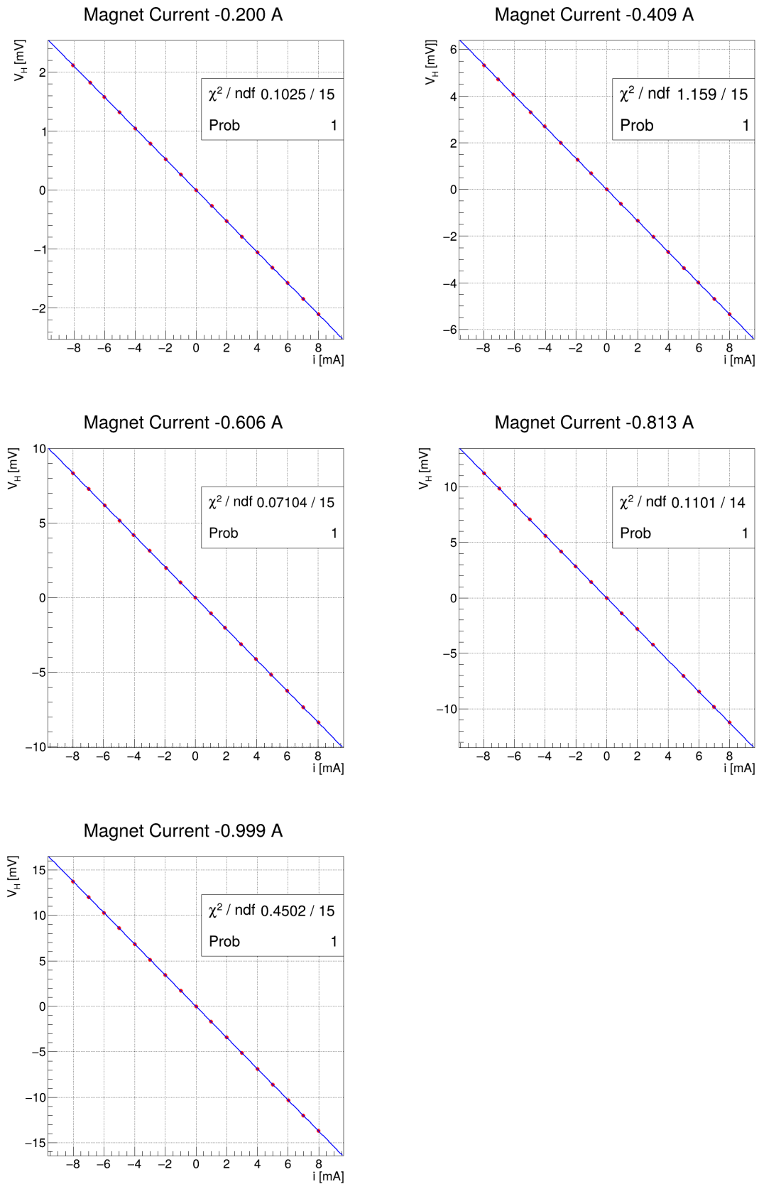
Fig. 3.3: Regressioni (in blu, con parametri dei fit in legenda) all'andamento della tensione di Hall V_H (in mV) contro la corrente nella sonda i_p (in mA) al variare del campo magnetico esterno (determinato dalla “magnet current” nel titolo, indicata più precisamente nel seguito).
