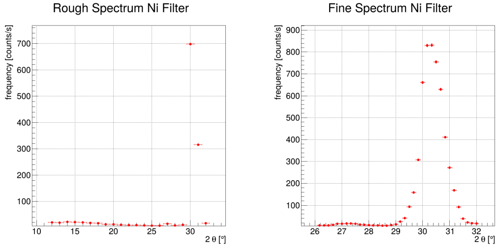
Fig. 4.2: Frequenze di rilevazione dei raggi X in \Delta t = 20\text{s} al variare dell'angolo (misurato in scala 2\theta ) di diffrazione del fascio sul cristallo di NaCl filtrato dal Ni. A sinistra i dati relativi alla scansione grossolana (con passo di 1^\circ ), mentre a destra quelli della scansione fine (con passo di 1/6^\circ ).
