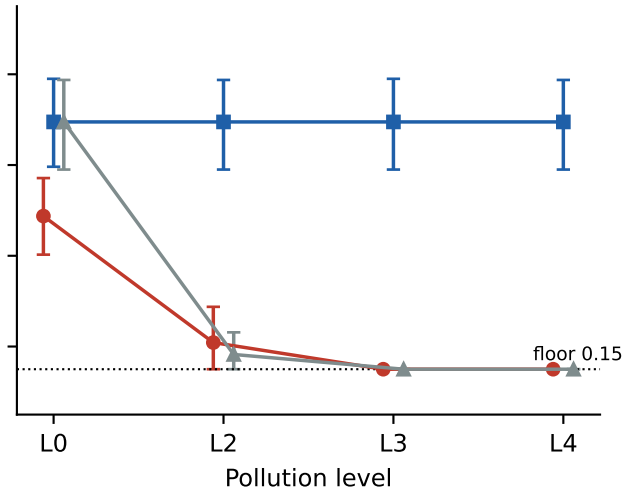
Gemma-3-4B-it (INT4)
