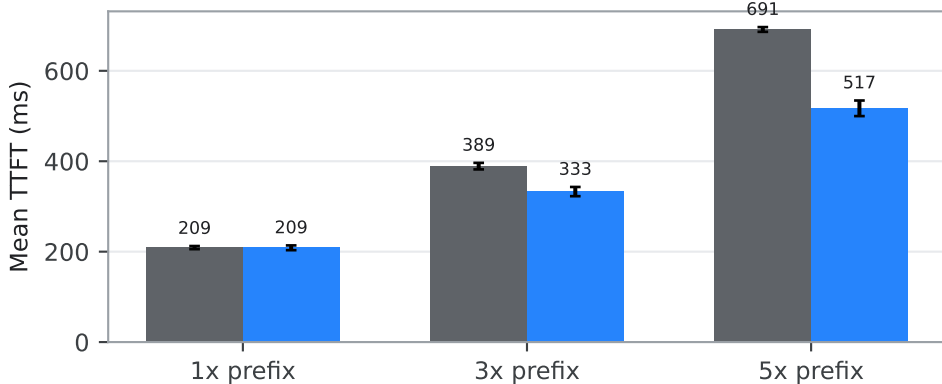
Qwen3-1.7B: Mean TTFT
