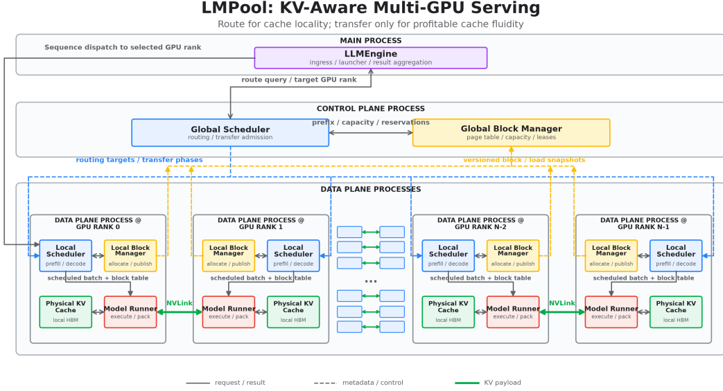
Figure 1: LMPool 的request、control、metadata 与KV data path 分别位于main process、control plane 和per-GPU data plane。每个详细GPU rank 使用相同的 2 \times 2 布局，重复rank pair 表示其他实例。Global Scheduler 向每个Local Scheduler 发送routing 和transfer command；每个Local Block Manager 向Global Block Manager 发布版本化block 与load snapshot。只有配对的Model Runner 通过绿色NVLink path 交换打包KV tensor，物理KV data 不经过control plane。
