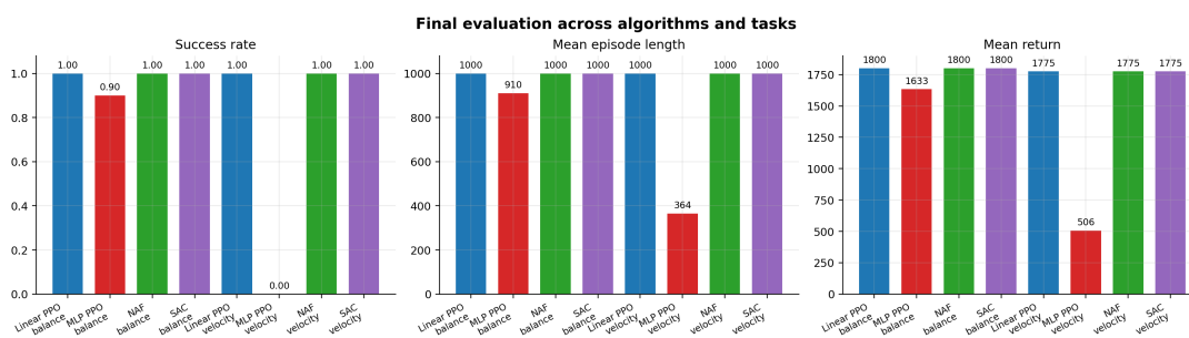
图 2 各方法最终评估指标
