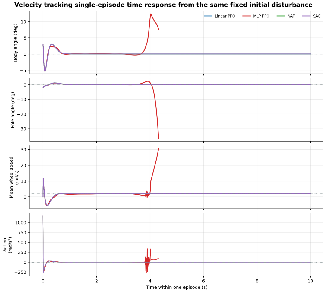
图 7 匀速跟踪任务的单回合动态响应
