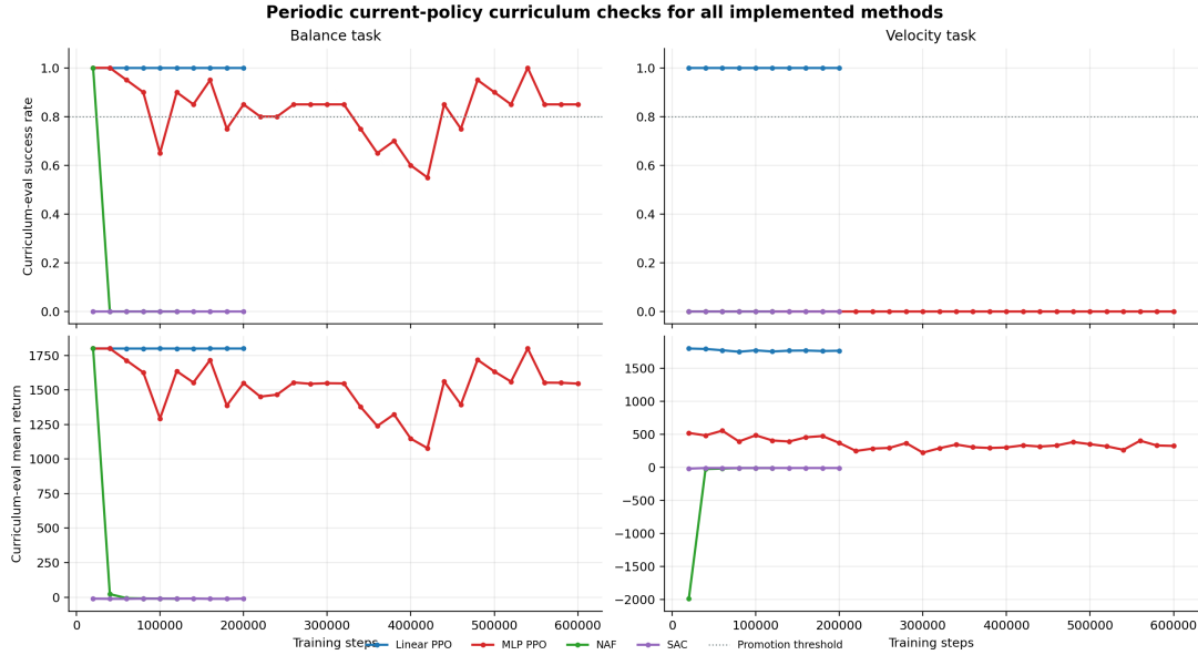
图 4 各方法课程训练过程中的周期评估结果
