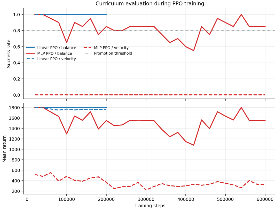
图 5 两种 PPO 策略的课程评估曲线
