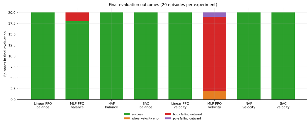
图 3 最终评估回合的结果分布
