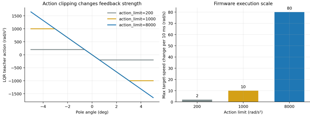
图 8 动作尺度对可用控制范围的影响
