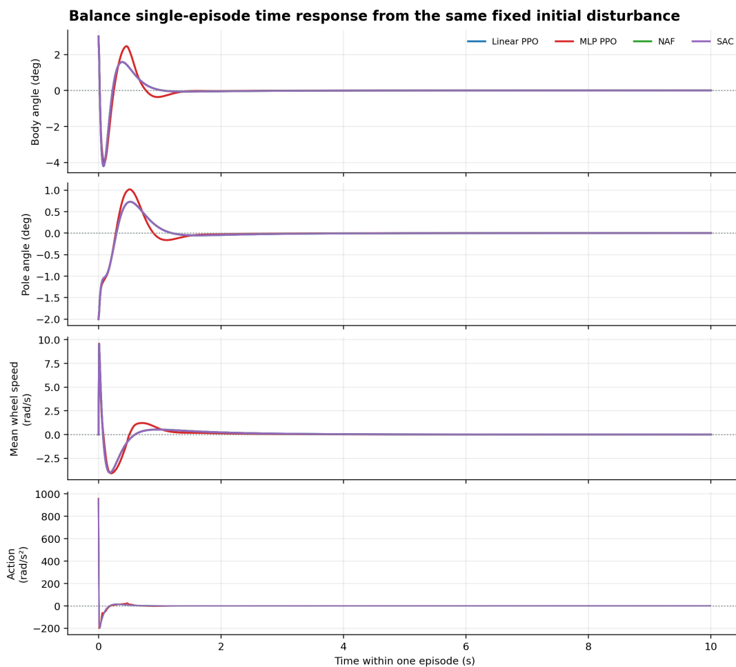
图 6 原地平衡任务的单回合动态响应
