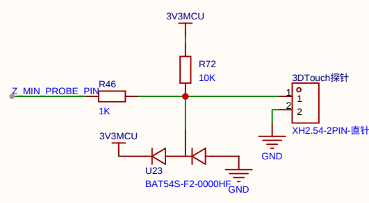
Z轴限位（3DTouch探针）
