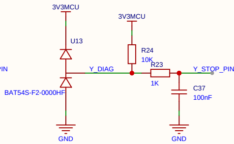
Y轴限位（DIAG无传感器回零）
