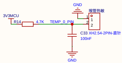
热端喉管温度传感器
