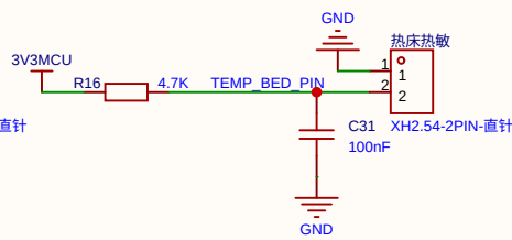
热床温度传感器
