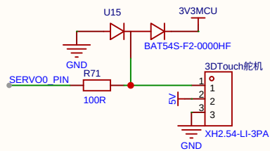
调平探头（3DTouch舵机）
