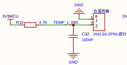
打印机舱体温度传感器
