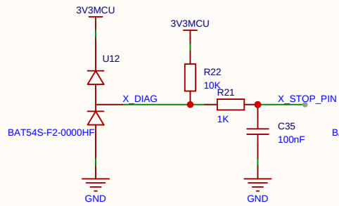
X轴限位（DIAG无传感器回零）
