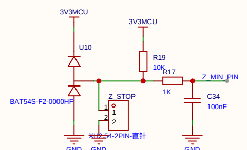
Z轴防撞保护（机械限位开关）
