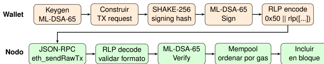
Figura 4.2: Flujo de una transacción post-cuántica: desde la generación de claves y firma en el wallet hasta la verificación e inclusión en un bloque en el nodo.
