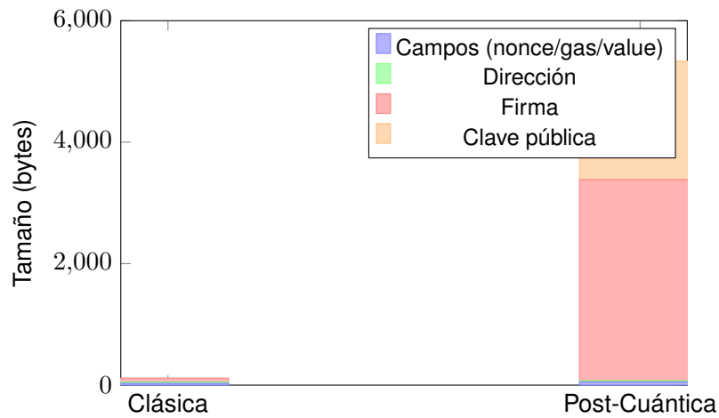
Figura 5.1: Comparativa de tamaño de transacción por componente. La firma ML-DSA-65 (3.309 B) y la clave pública (1.952 B) constituyen el 99 % del incremento.
