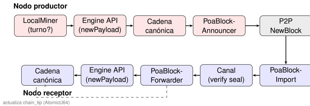
Figura 4.3: Propagación de bloques PoA: el nodo productor anuncia el bloque vía P2P; el nodo receptor lo importa, verifica el sello ML-DSA-65 y lo inyecta en su cadena canónica mediante la engine API.
