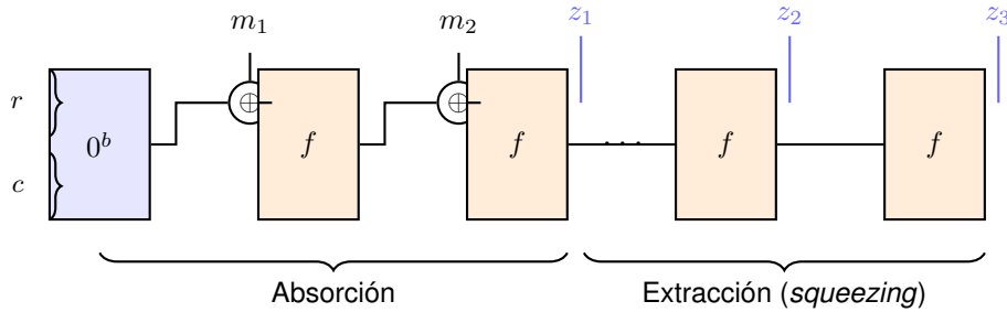
Figura 2.3: Construcción esponja: los bloques del mensaje m_i se absorben mediante XOR con la tasa r del estado seguido de la permutación f . En la fase de extracción, se extraen r bits por aplicación de f . La capacidad c nunca se expone directamente.
