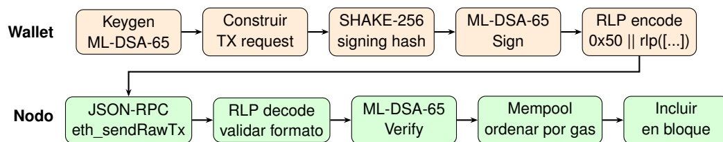
Figura 4.1: Flujo de una transacción post-cuántica: desde la generación de claves y firma en el wallet hasta la verificación e inclusión en un bloque en el nodo.
