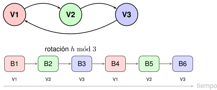
Figura 4.2: Rotación round-robin de 3 validadores: cada bloque h es producido por el validador h \bmod 3 , garantizando una distribución equitativa.
