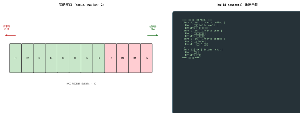
图 7: 记忆系统滑动窗口示意图。左侧为 maxlen=12 的 deque 结构, 右侧为 build_context() 生成的格式化文本块示例。
