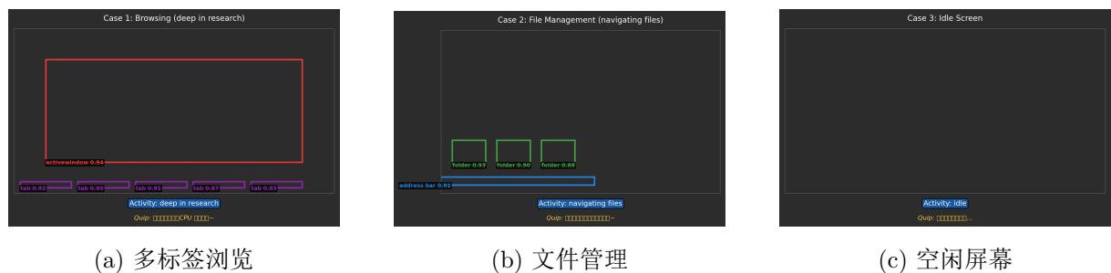
图 11: YOLOv8 在三种典型桌面场景下的 UI 元素检测结果。
