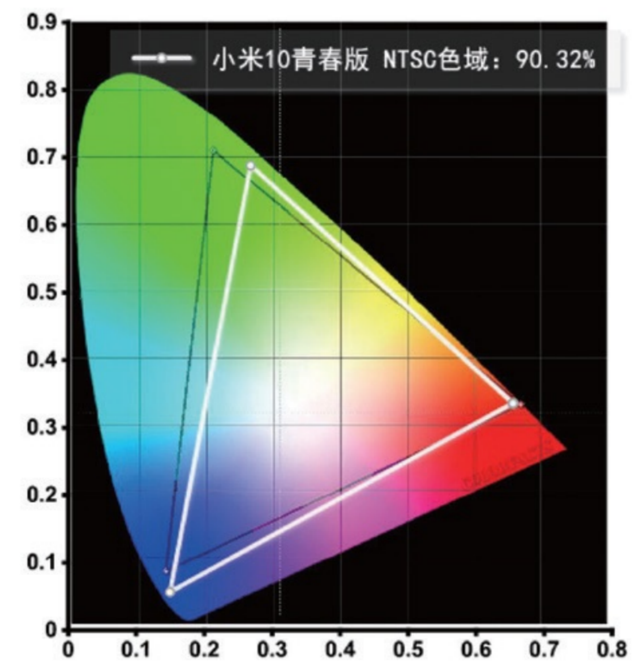
▲实测屏幕覆盖90.32%的NTSC色域，色彩鲜艳丰富。
