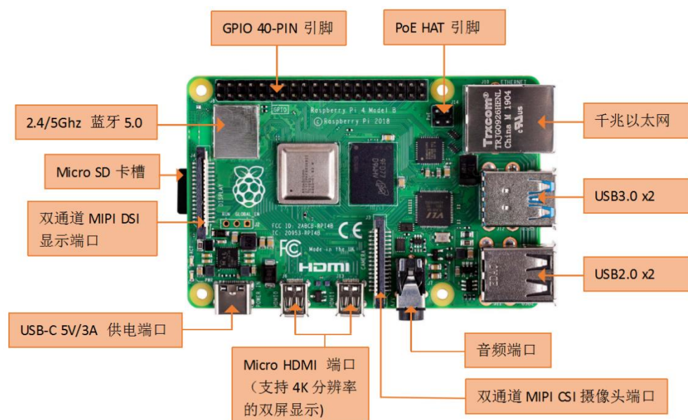
树莓派 4 的引脚和接口说明
