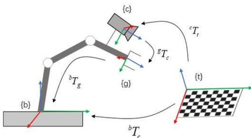
手眼标定示意图
