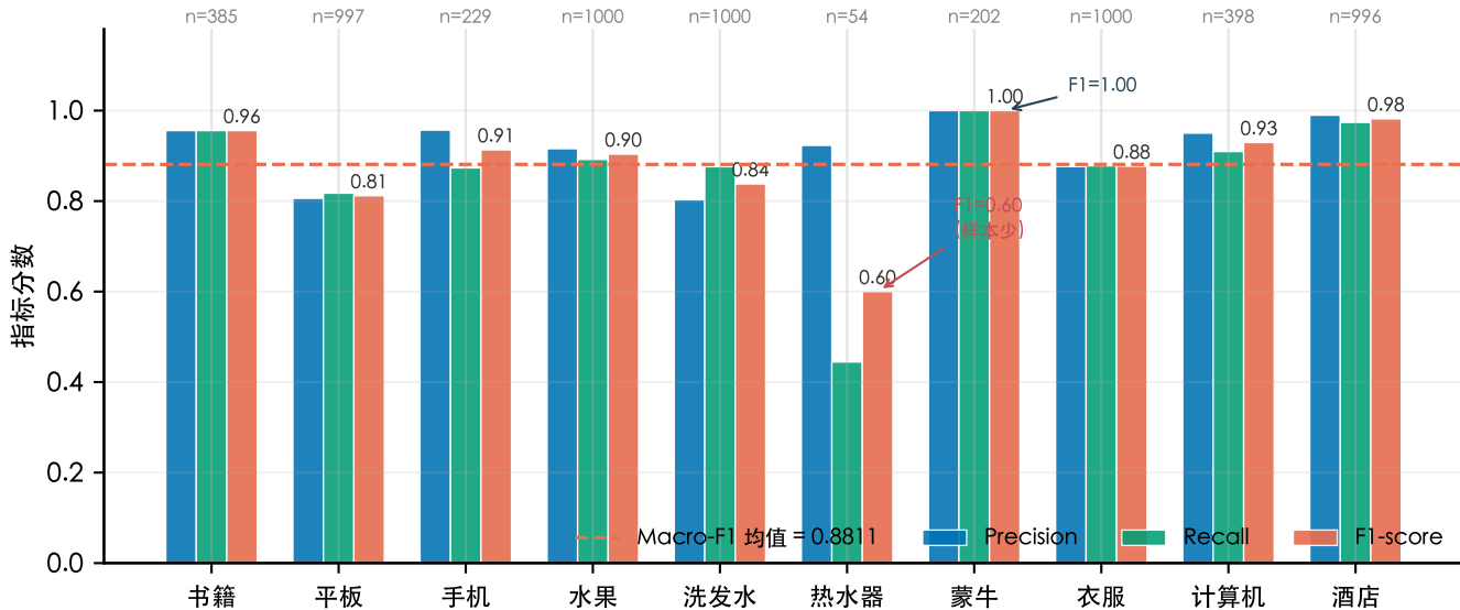
图3 各类别 Precision / Recall / F1 对比（测试集）
