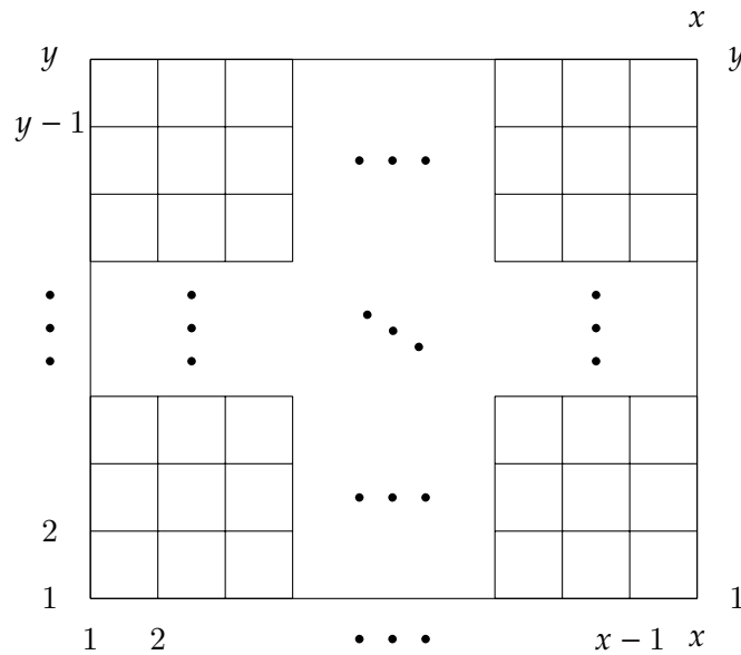
Figura 3.1 – Tablero de Go de dimensiones x \times y .
