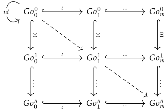
Figura 3.11 – Estructura de la familia de Juegos de Go . A derecha agregamos jugadores, hacia abajo expandimos el tablero.
