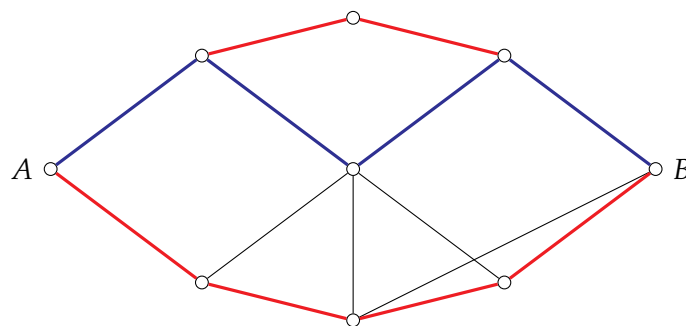
Figura 3.16 – Las aristas azules pertenecen a Short, las rojas a Cut y las negras permanecen libres. El conjunto de aristas azules determina un camino entre los vértices distinguidos A y B , por lo que Short gana.
