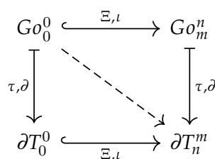
Figura 3.12 – Diagrama de la estructura completa. Las flechas horizontales ( \Xi ) expanden dimensiones y jugadores ( l ). Las verticales ( \tau ) cierran el espacio y ( \partial ) vacían el interior.
