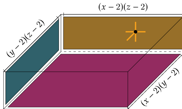
Figura 3.3 – Caras del tablero de tres dimensiones con un nodo de 5 adyacencias.
