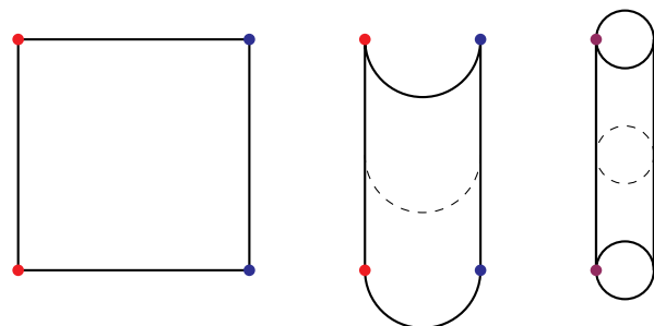
Figura 3.5 – Transición del plano a cilindro al unir sus lados opuestos.
