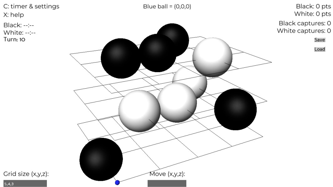
Figura 3.4 – Tablero de 5 \times 4 \times 3 en 3dGo .
