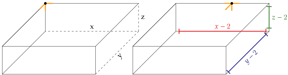
Figura 3.2 – Exterior del tablero tres dimensional. Un vértice con 3 adyacencias, aristas y un nodo con 4 adyacencias.
