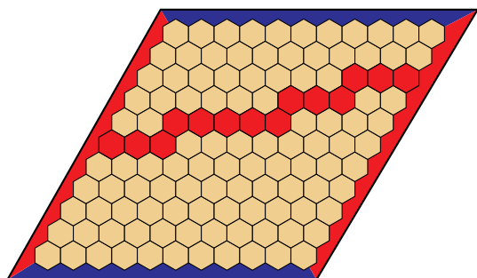
Figura 3.15 – Cadena ganadora que conecta dos bordes opuestos.
