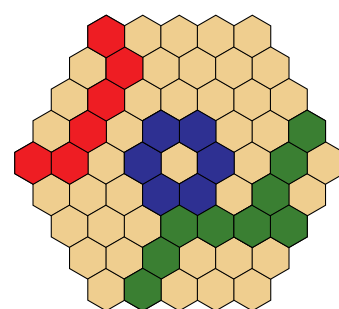
Figura 3.14 – Las tres estructuras ganadoras en el Havannah: anillo , punto y tenedor .
