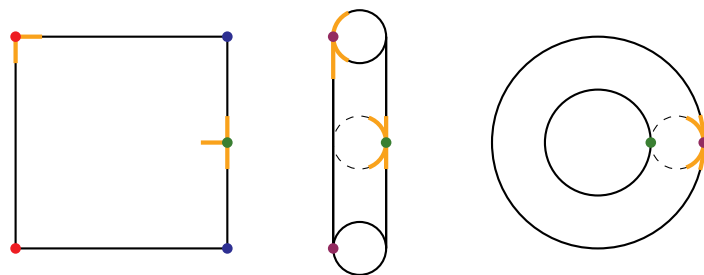
Figura 3.7 – Cambio de las adyacencias desde el plano al toro.
