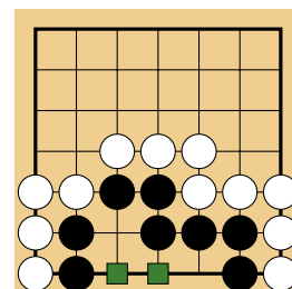
Figura 2.15 – Tablero con grupos negros cuya región controlada es no saludable .
