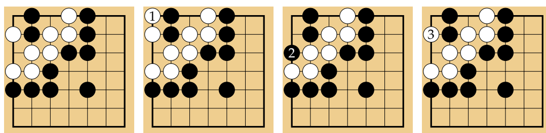
Figura 2.7 – Tablero con un ciclo de tres jugadas.
