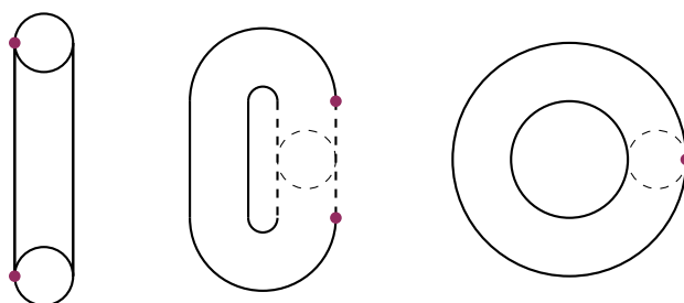
Figura 3.6 – Transición del cilindro al toro tras unir sus caras opuestas.
