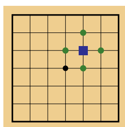
Figura 2.1 – Punto (5, 5) en azul, adyacencias en verde.
