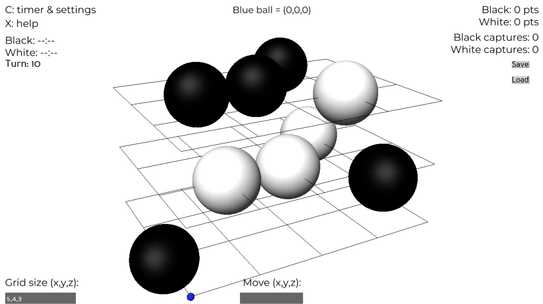
Figure 3.4 – Tablero de 5 \times 4 \times 3 en 3dGo .
