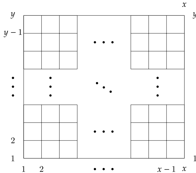
Figure 3.1 – Tablero de Go de dimensiones x \times y .
