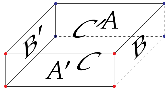
Figura 3.8 – Caras del Go^3 .
