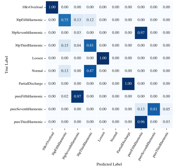
(d) ConvNeXt-Tiny
