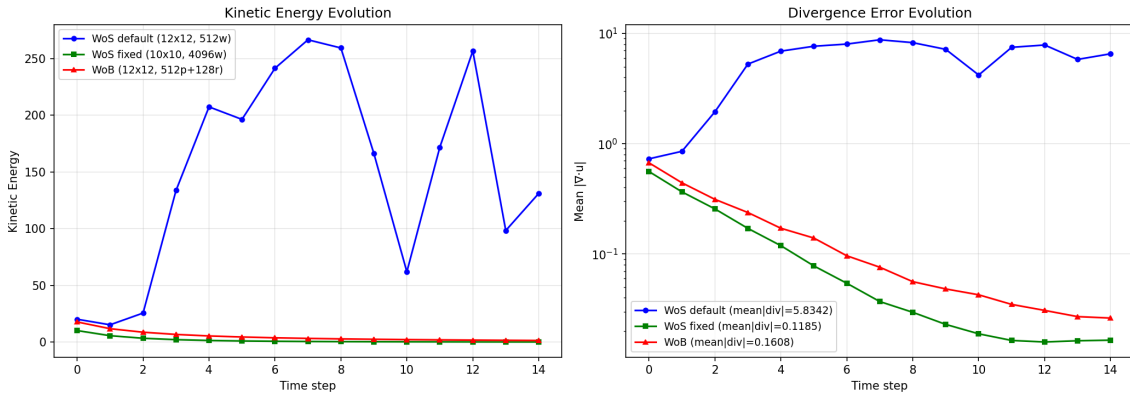
Figure 4: 三种方案的动能与散度误差演化对比。（ \Delta t = 0.03 , \nu = 0.05 。WoS 默认: 12 \times 12 网格, N_{\text{walk}} = 512 ; WoS 修复: 10 \times 10 网格, N_{\text{walk}} = 4096 , \sigma = 0.5 ; WoB: 12 \times 12 网格, N_{\text{part}} = 512 , N_{\text{ray}} = 128 ）
