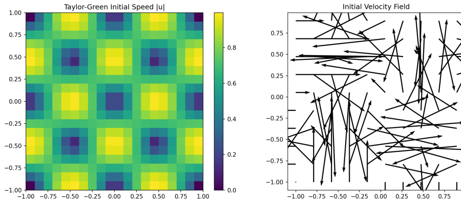
Figure 1: Taylor-Green 衰减涡初始条件：速度大小场（左）与矢量场（右），网格分辨 20 \times 20 。
