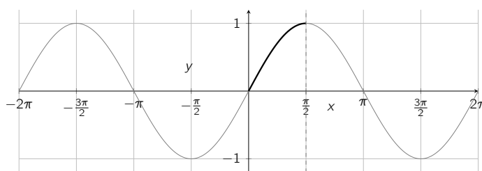
Représentation graphique de la fonction sinus
