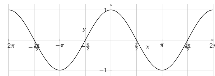
Représentation graphique de la fonction cosinus
