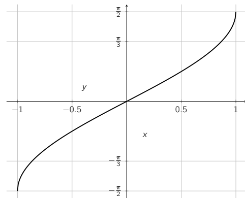
Représentation graphique de la fonction arc sinus
