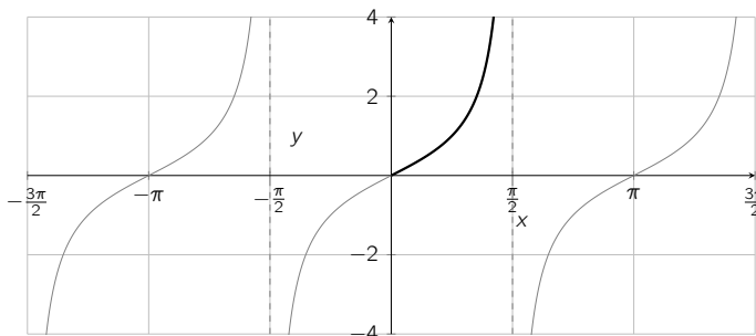
Représentation graphique de la fonction tangente
