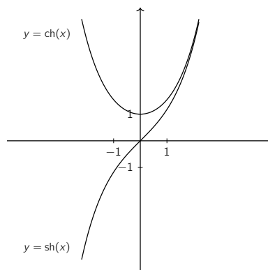
Représentation graphique des fonctions hyperboliques
