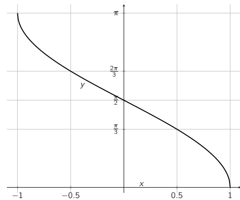
Représentation graphique de arc cosinus
