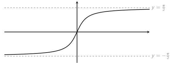
Représentation graphique de la fonction arc tangente
