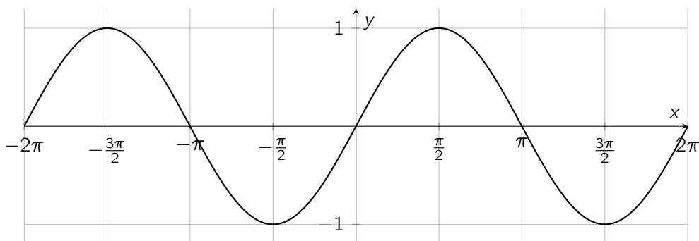
Représentation graphique de la fonction sinus
