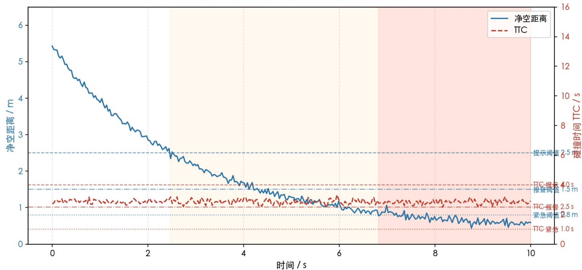
动态场景TTC-净空距离联合演化曲线（相向接近工况）
