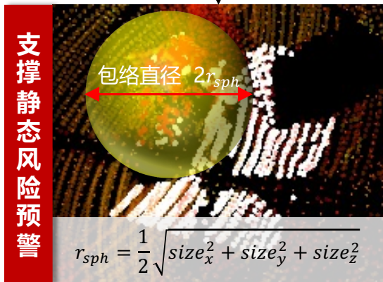
包络球生成
