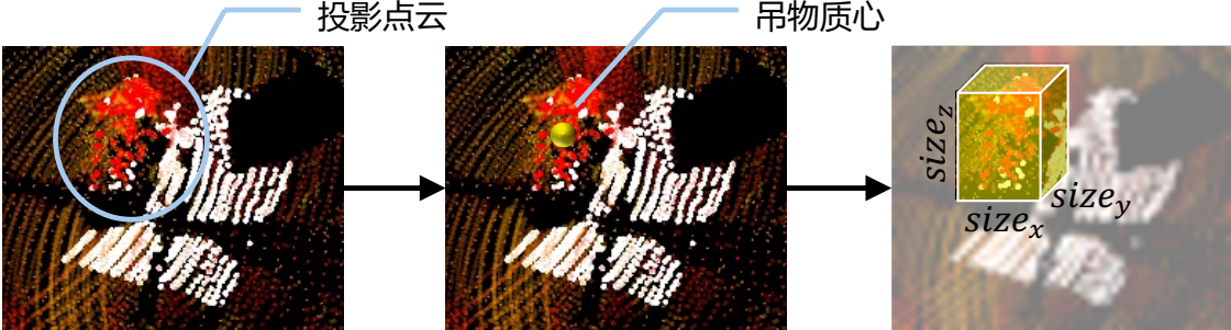
点云输入
