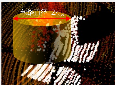
吊装构件-包络圆柱+状态
