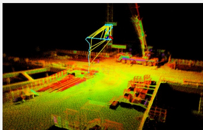
调平后配准点云+吊钩位姿
