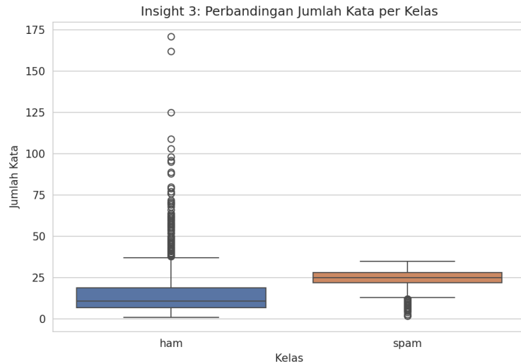
Gambar 3.3 Perbandingan Jumlah Kata per Kelas
