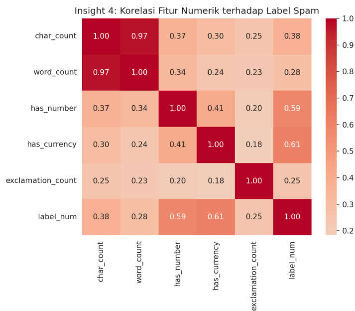
Gambar 3.4 Korelasi Fitur Numerik terhadap Label Spam
