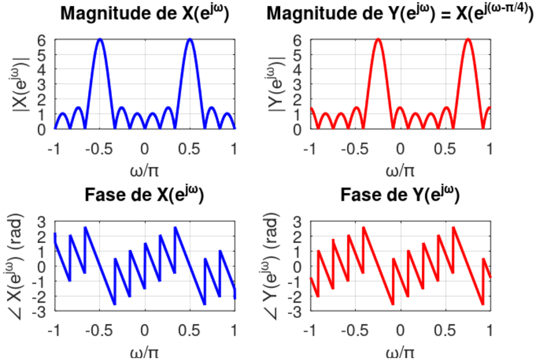
Figura 4 – Verificação da propriedade de deslocamento em frequência: magnitude e fase de X(e^{j\omega}) e Y(e^{j\omega}) .
