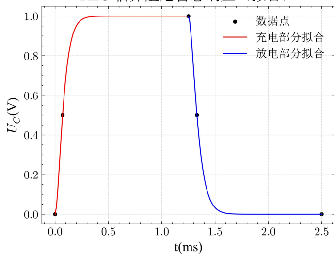
RLC 临界阻尼暂态响应（拟合）
