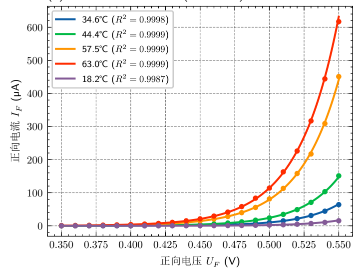
(b) PN 结伏安特性曲线 (线性坐标)
