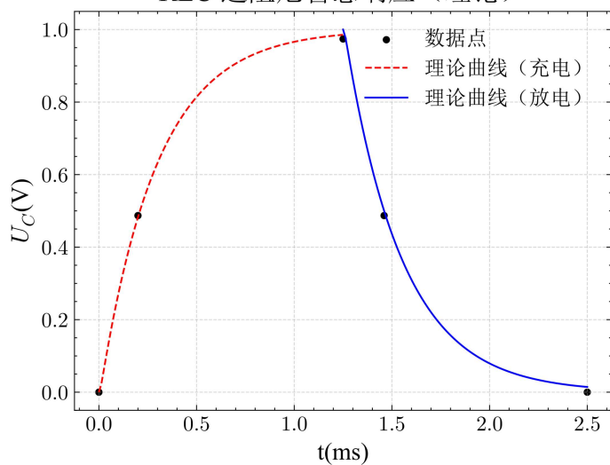
RLC 过阻尼暂态响应（理论）
