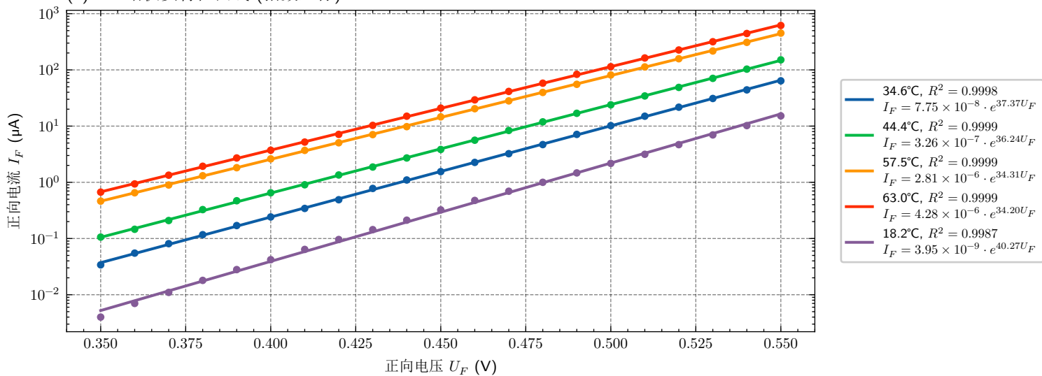
(a) PN 结伏安特性曲线 (指数坐标)
