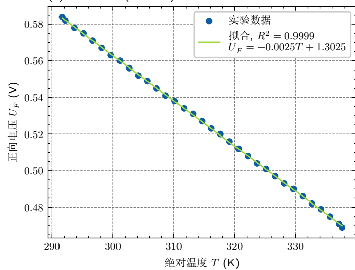
(c) U-T 关系 (第 1 组)
