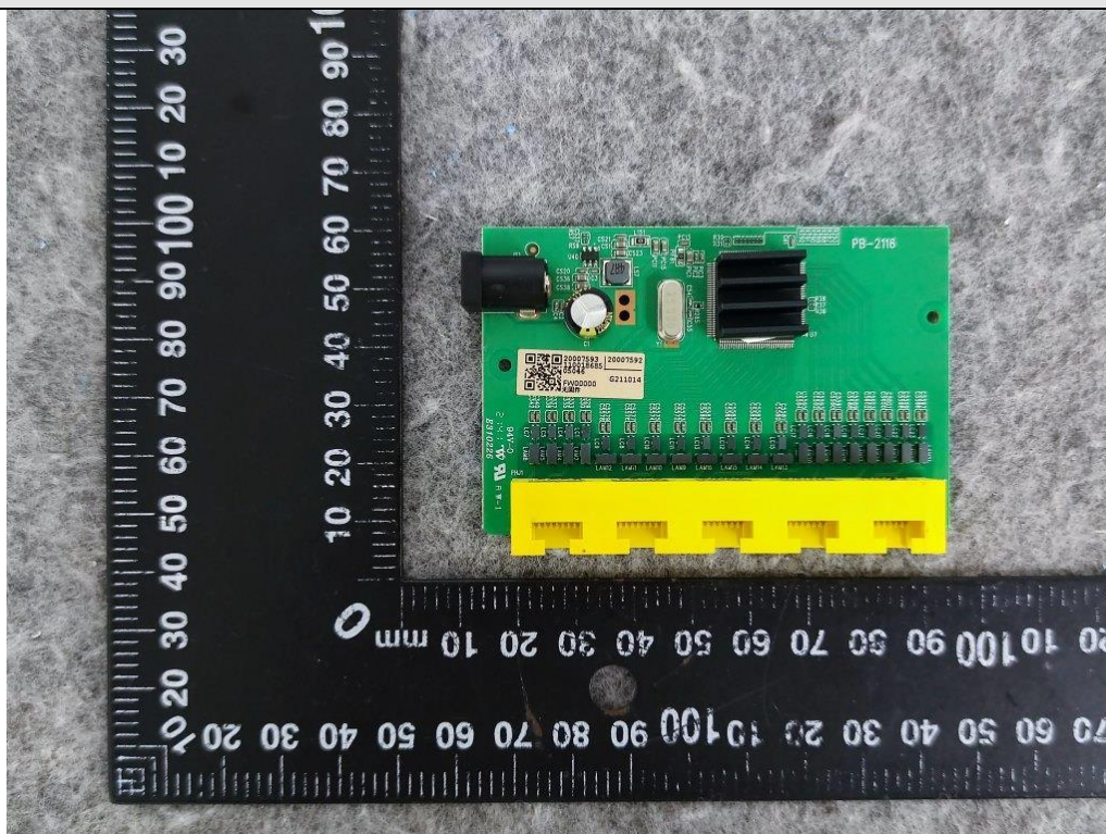
图7 主板正面
