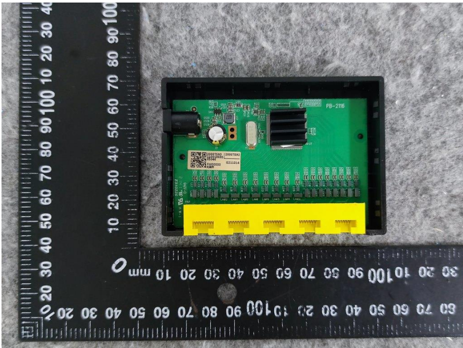
图1 内部结构
