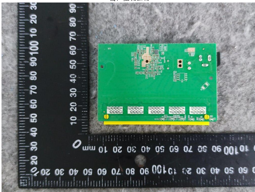
图8 主板背面
