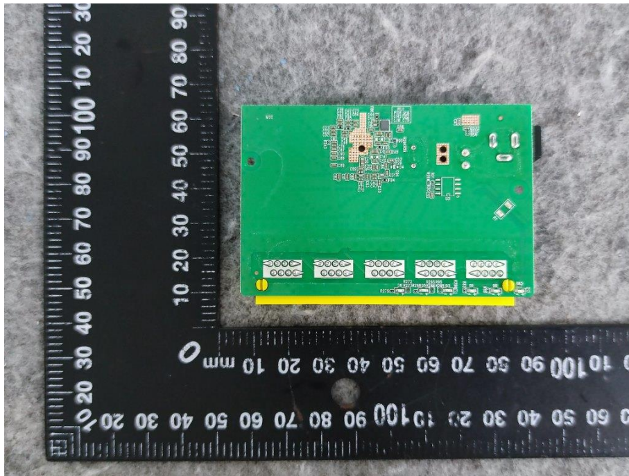
图3 主板反面
