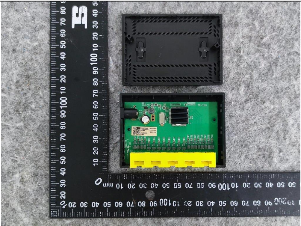
图5 内部结构
