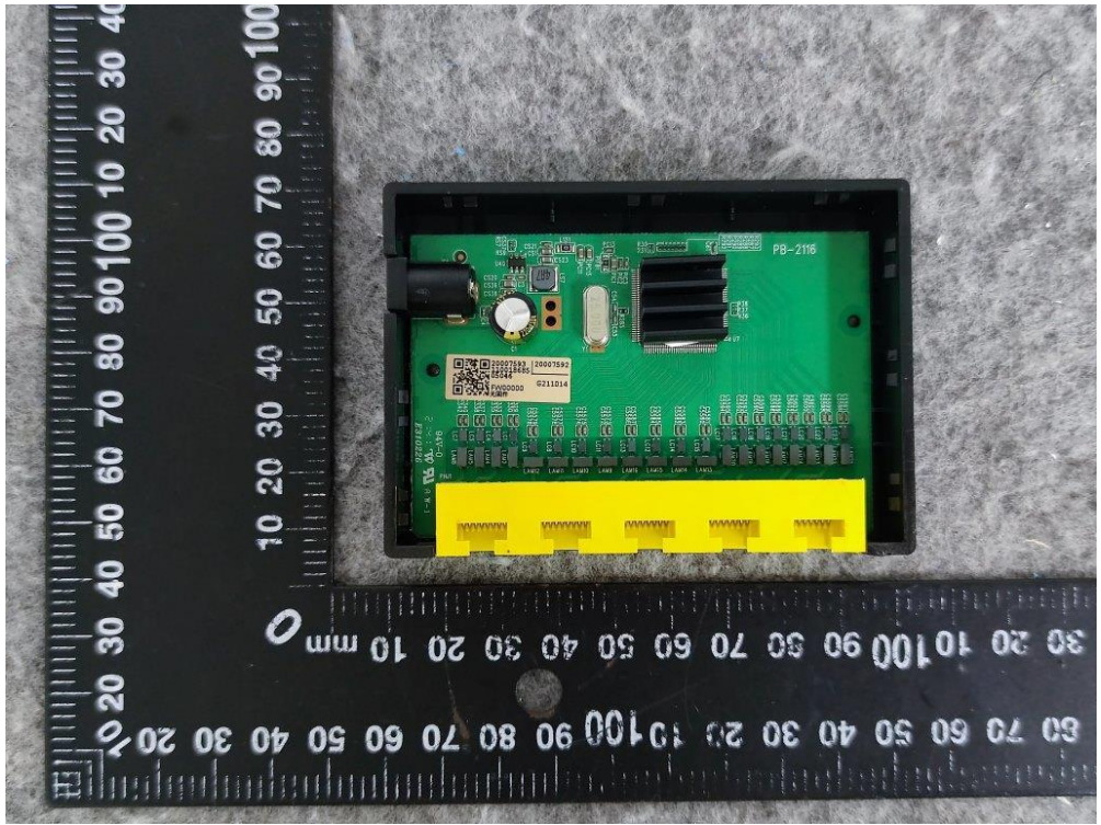
图6 内部结构
