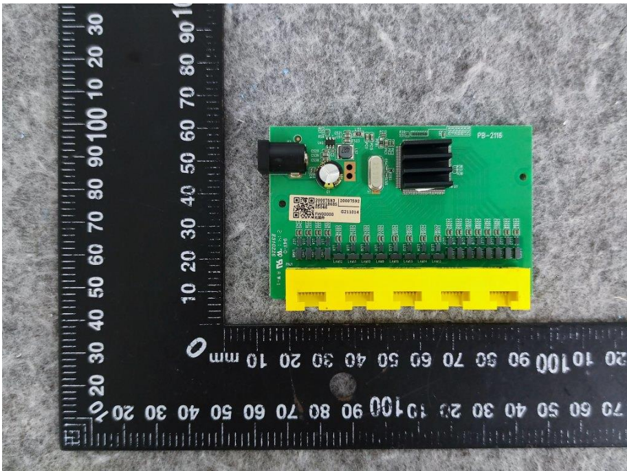
图2 主板正面
