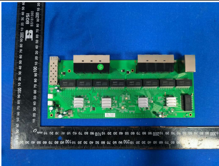
图五 内部结构
