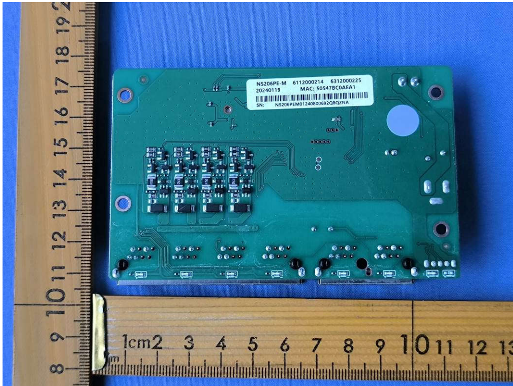
图九 产品内部控制板
