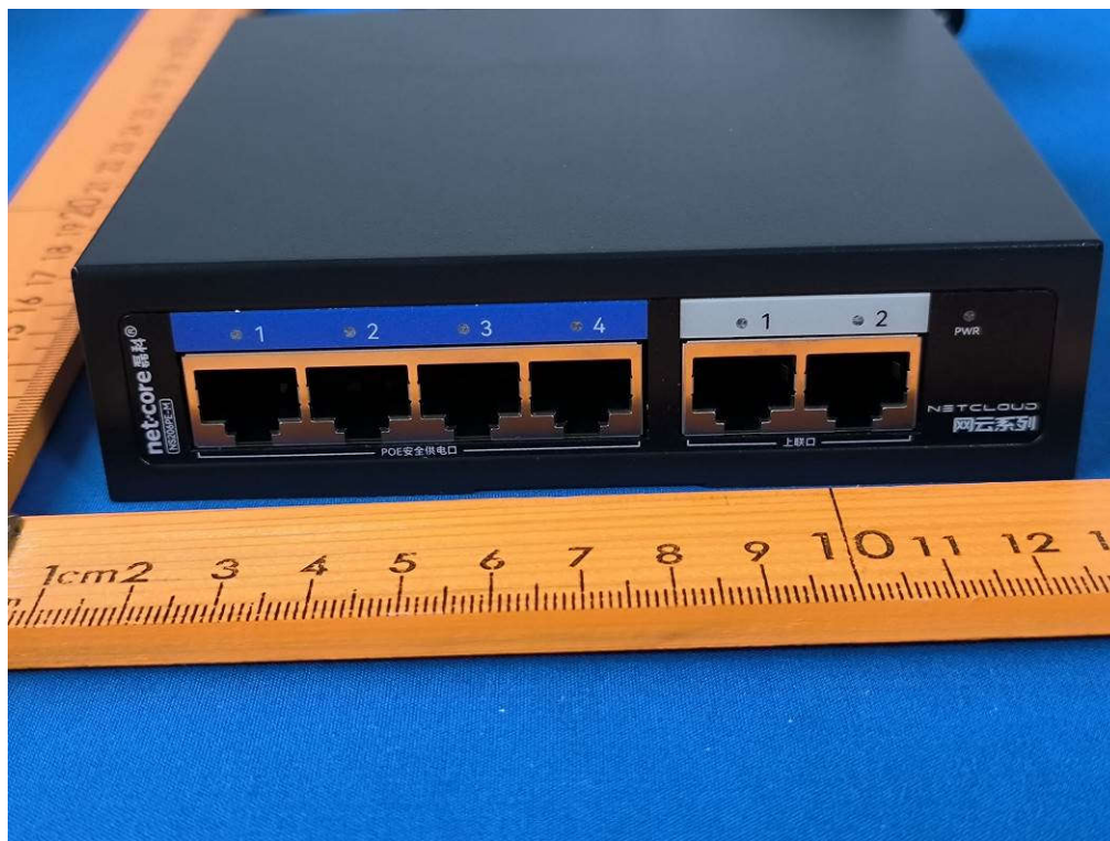
图三 产品外观
