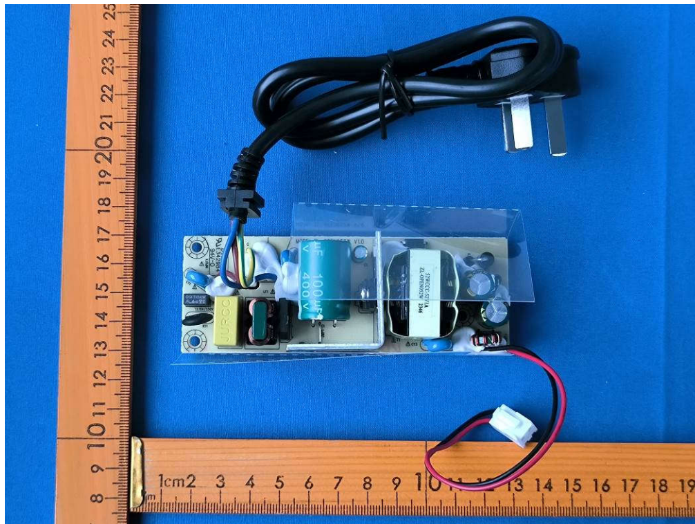
图七 产品内置电源
