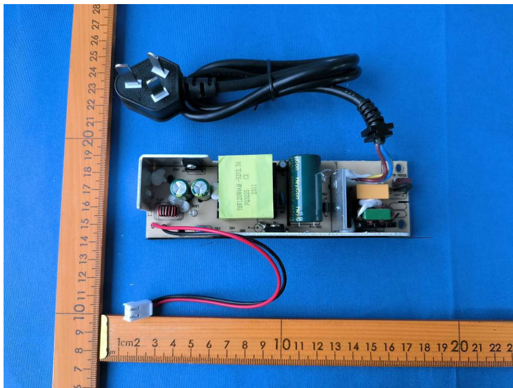
图六 产品内置电源
