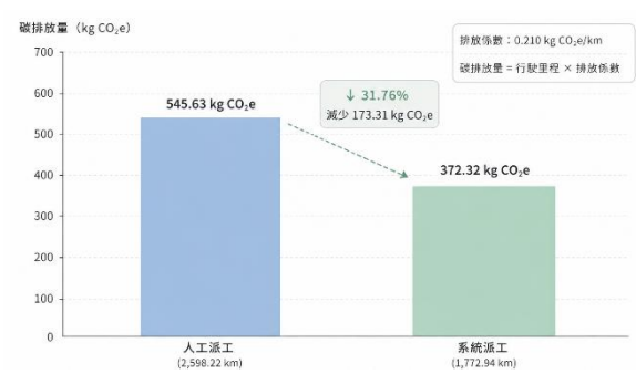
圖 3 人工派工與系統派工碳排放比較圖
