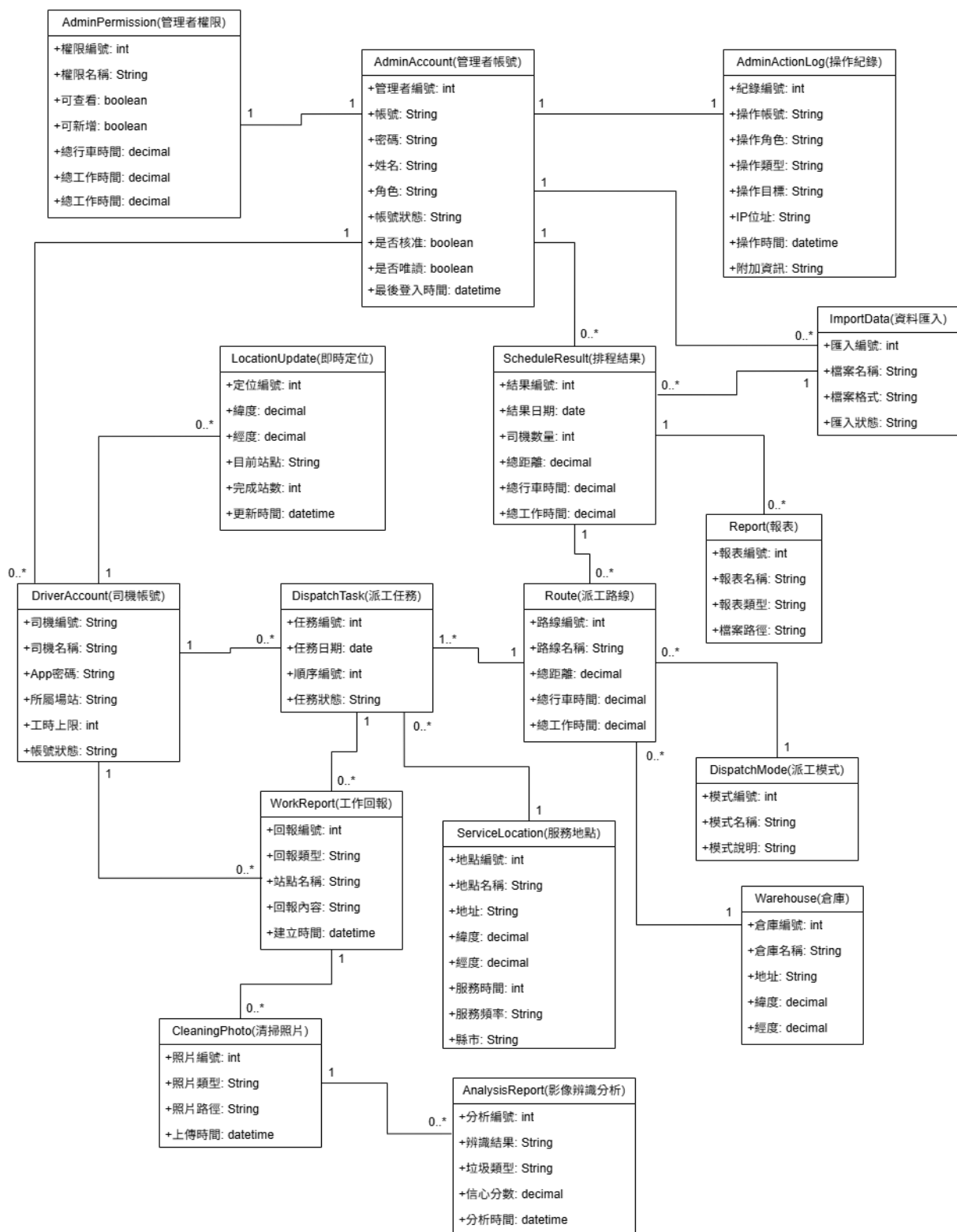
圖 5-4-1 分析類別圖
