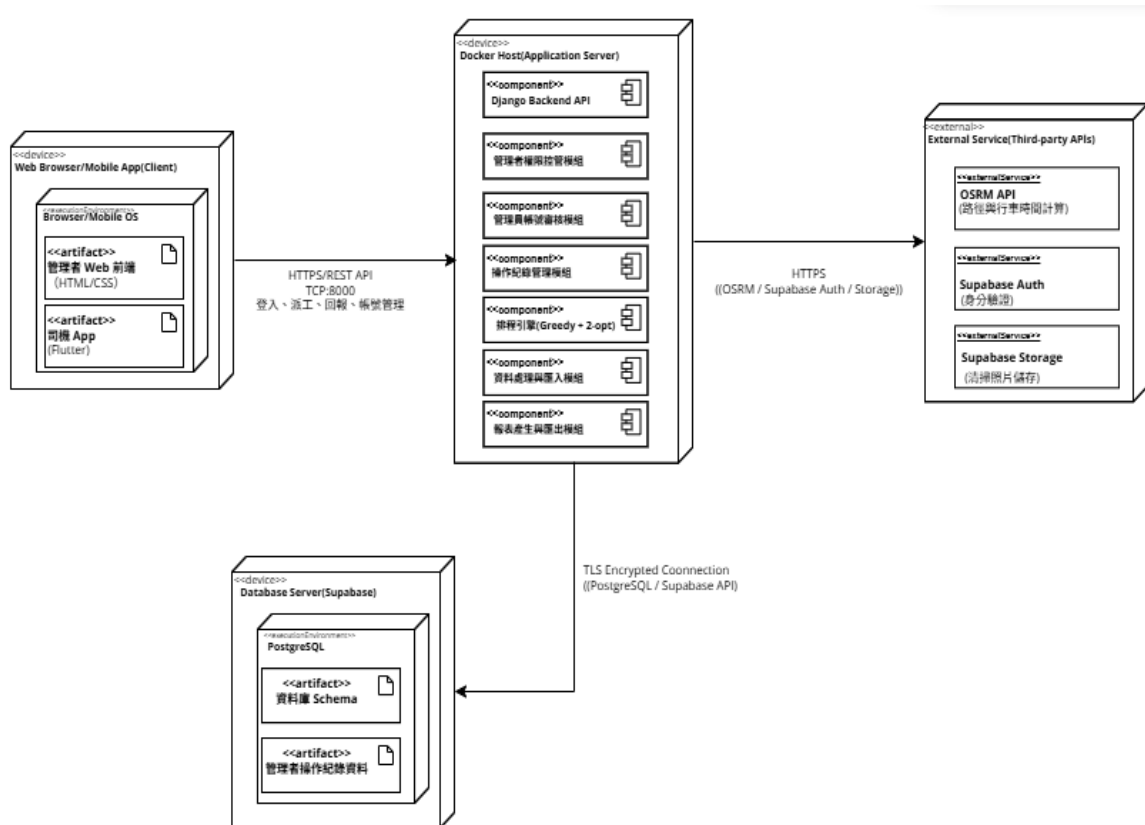
圖 7-1-1 佈署圖
