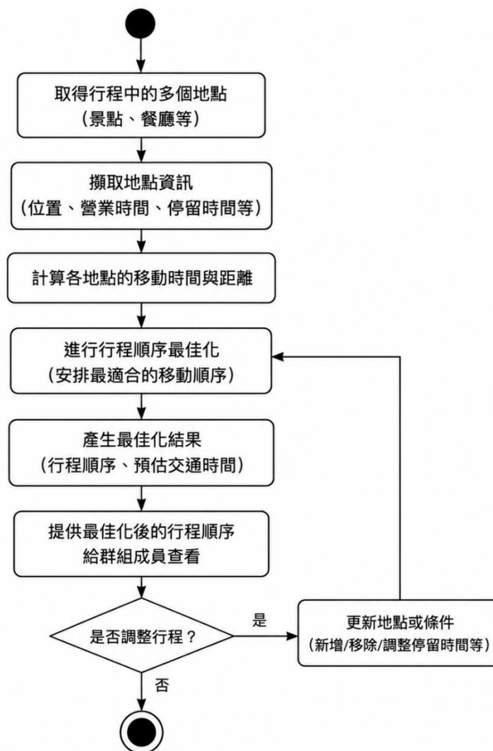
▲ 圖 5-3-5 行程順序最佳化活動圖
