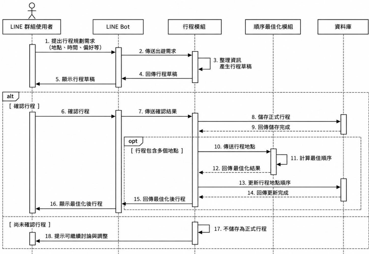
▲圖 6-1-4 行程規劃與順序最佳化循序圖 14
