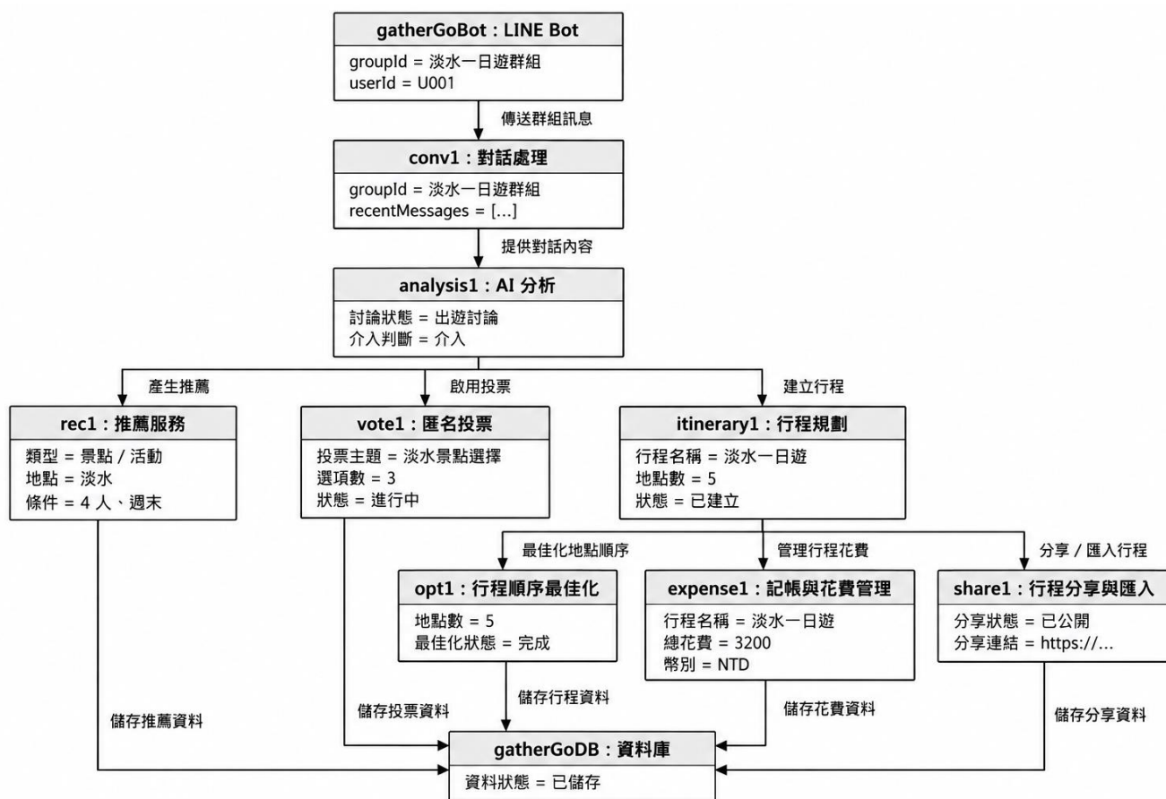
▲圖 6-2-2 設計物件圖 16
