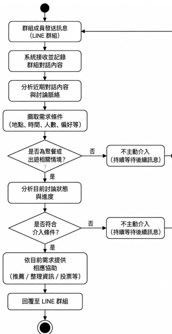
▲圖 5-3-1 群組對話分析與智慧介入活動圖 4
