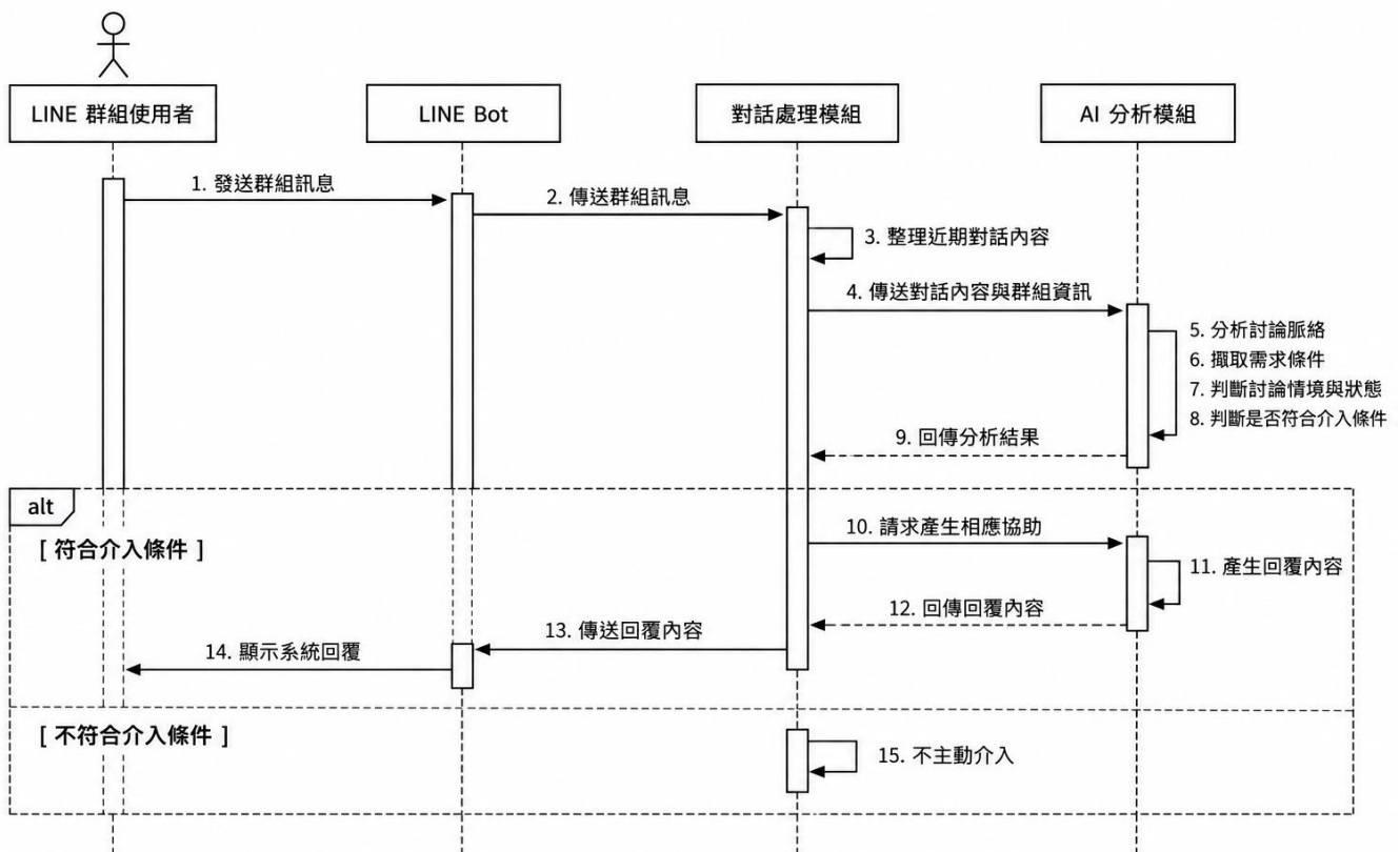
▲圖 6-1-1 群組對話分析與智慧介入循序圖 11
