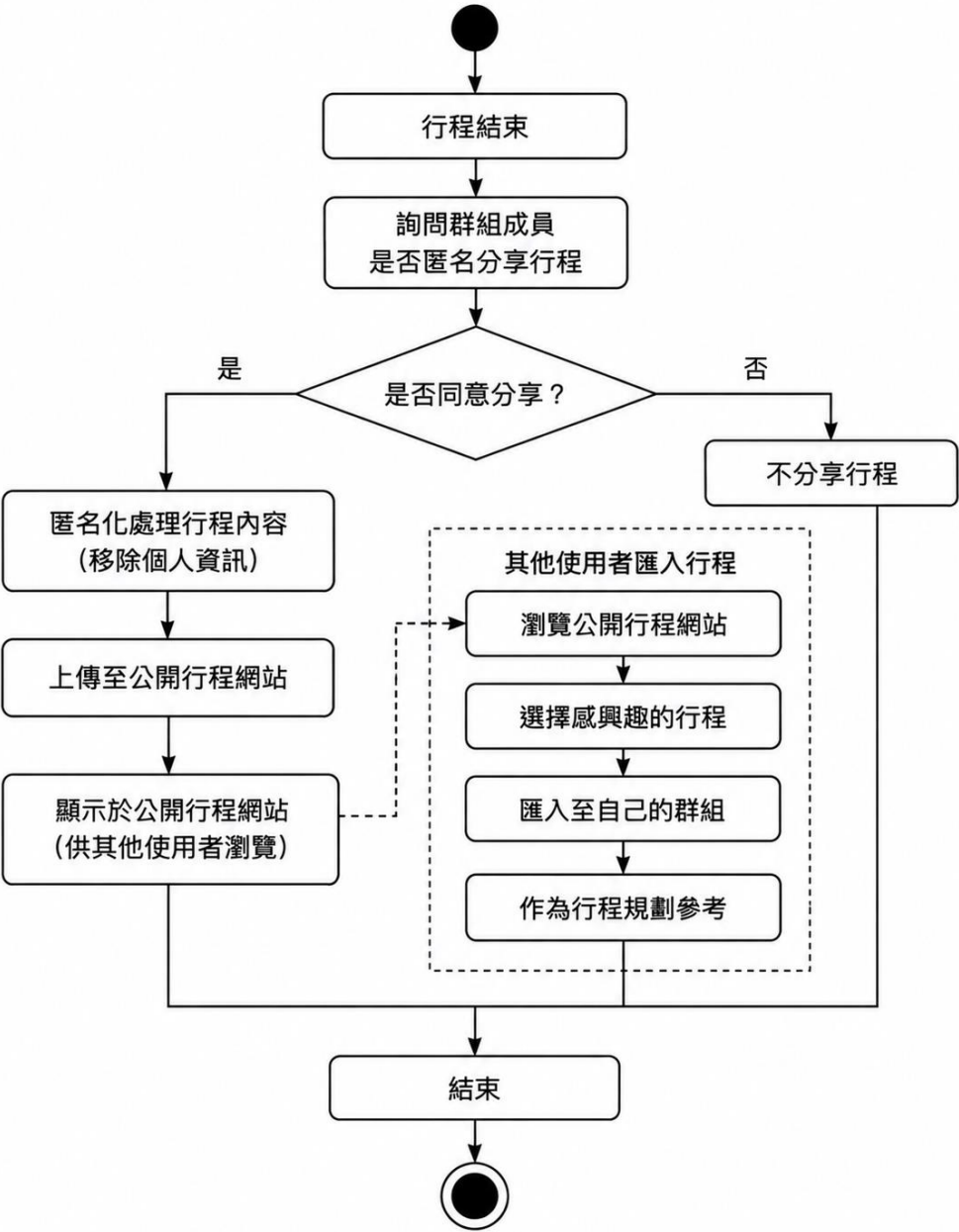
▲圖 5-3-7 行程分享與匯入活動圖
