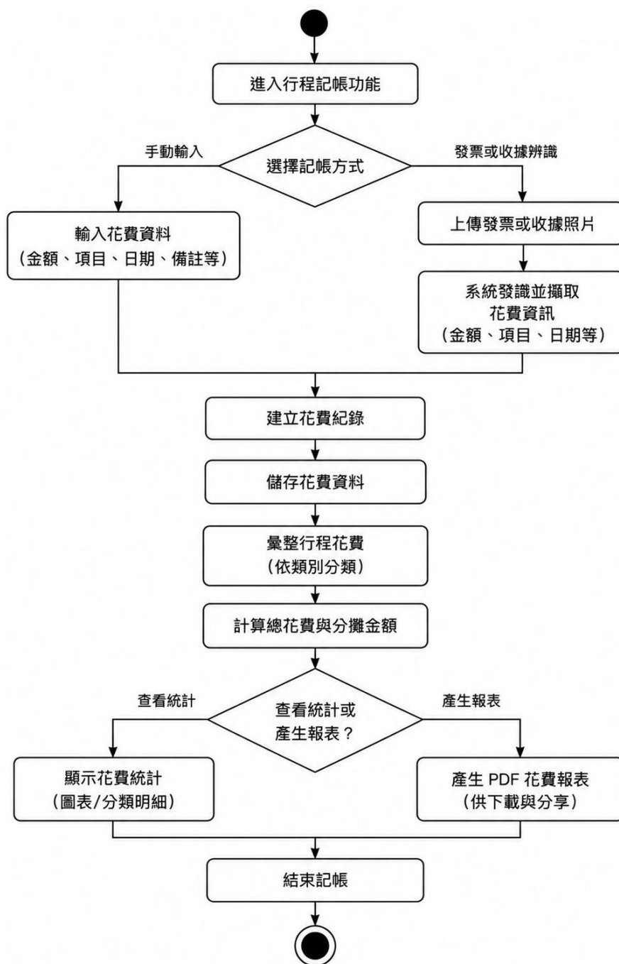
▲ 圖 5-3-6 記帳與花費管理活動圖
