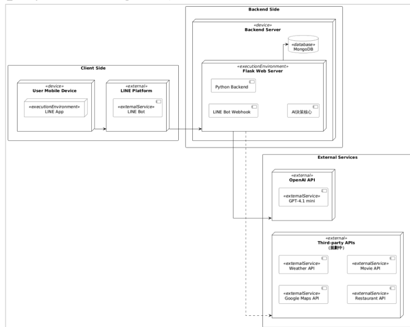
▲圖 7-1-1 佈署圖 17
