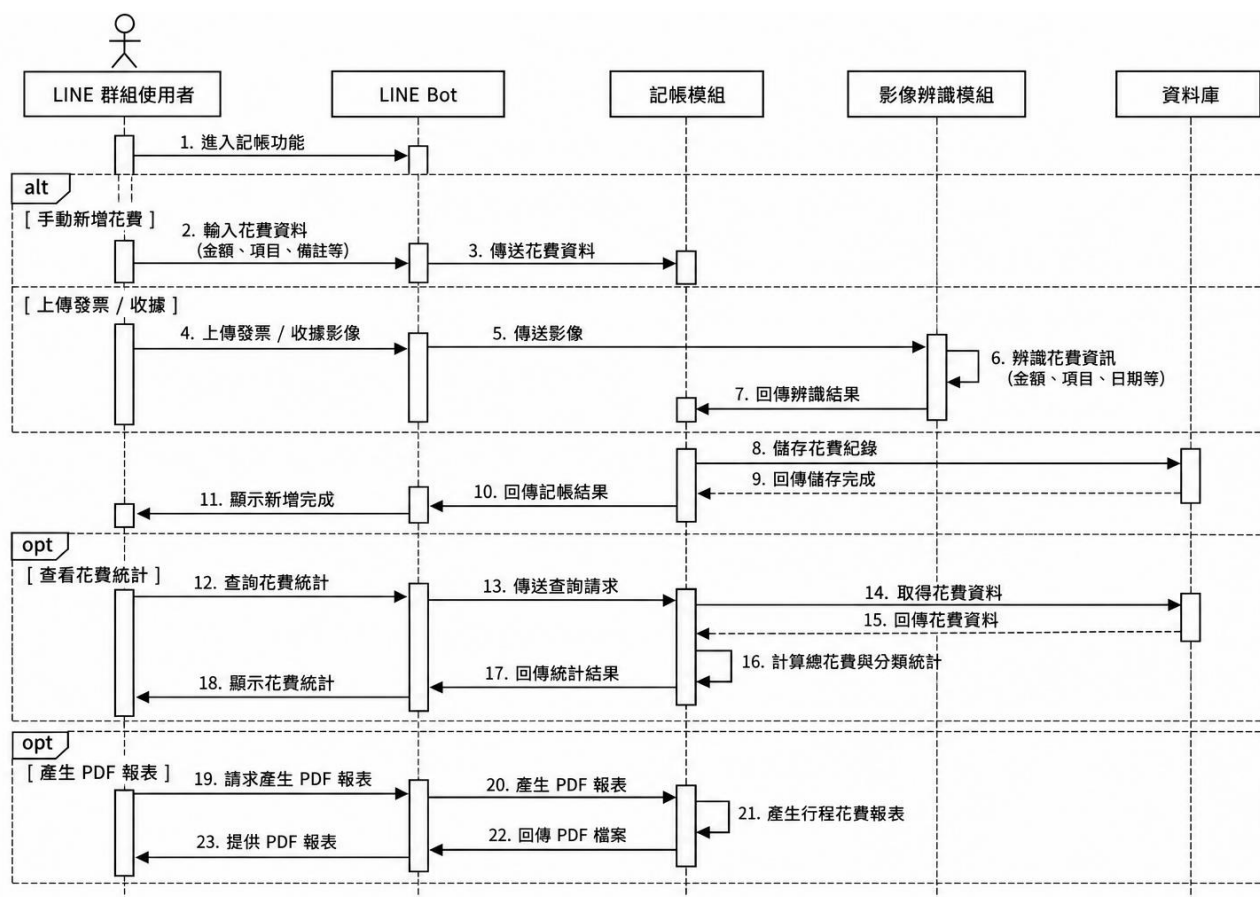
▲圖 6-1-5 記帳與花費管理循序圖
