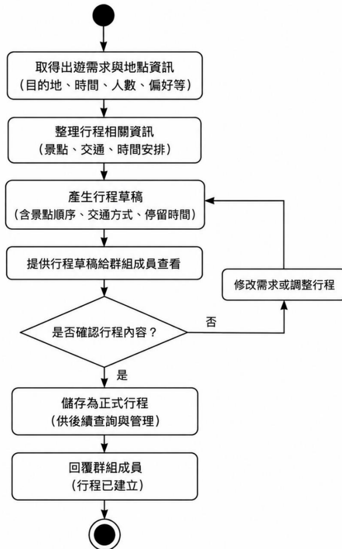
▲ 圖 5-3-4 行程規劃活動圖
