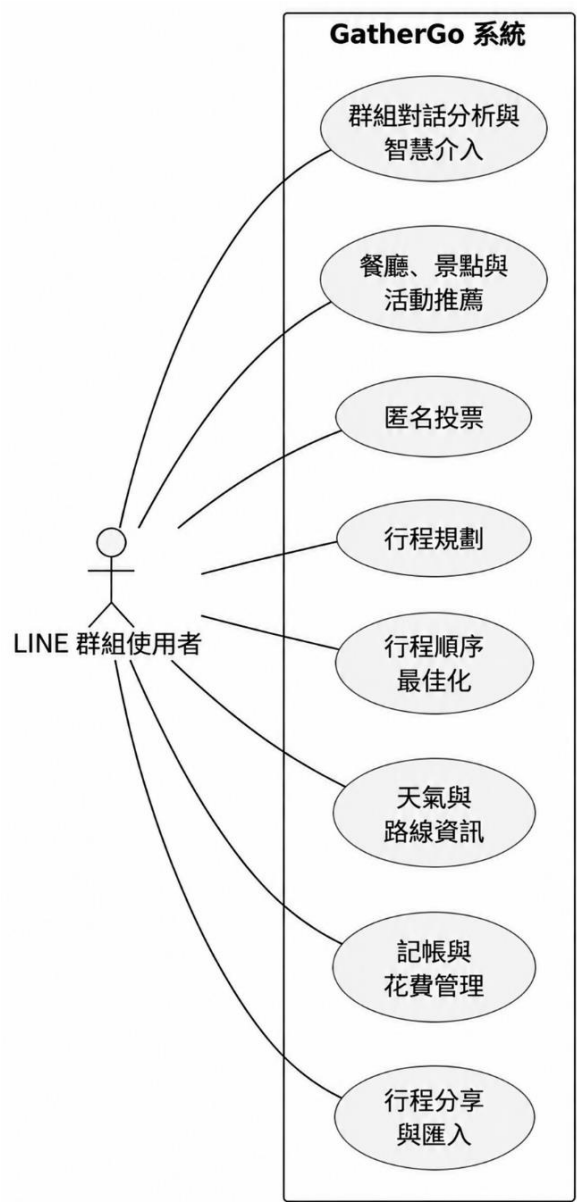
▲圖 5-2-1 使用個案圖 3
