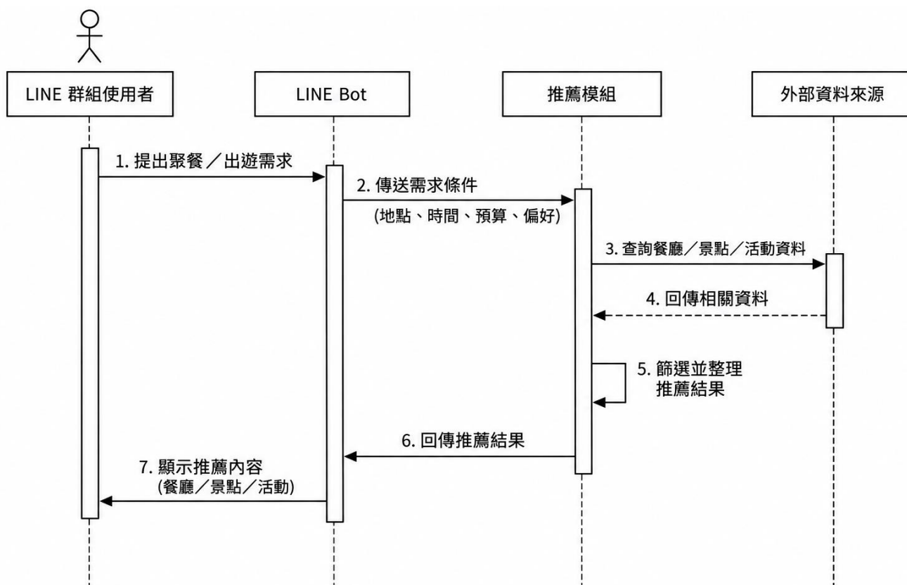
▲圖 6-1-2 餐廳、景點與活動推薦循序圖 12
