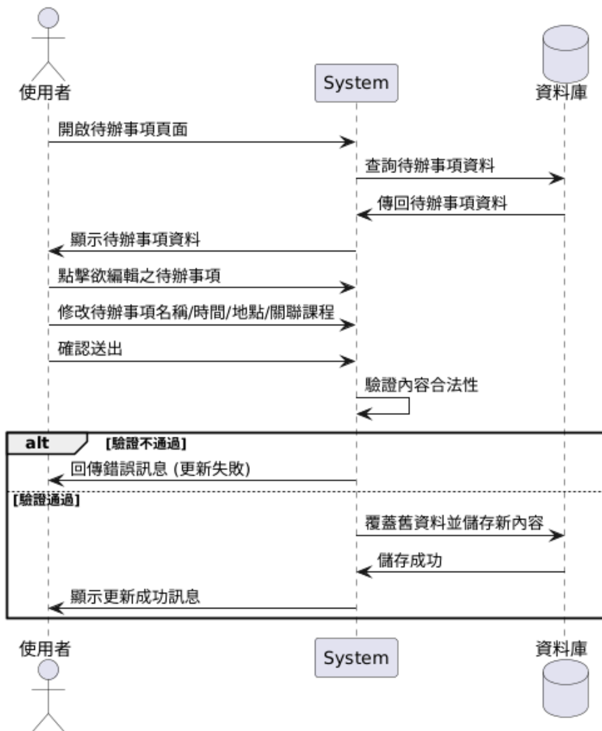
圖 6-1-7 循序圖之編輯待辦事項
