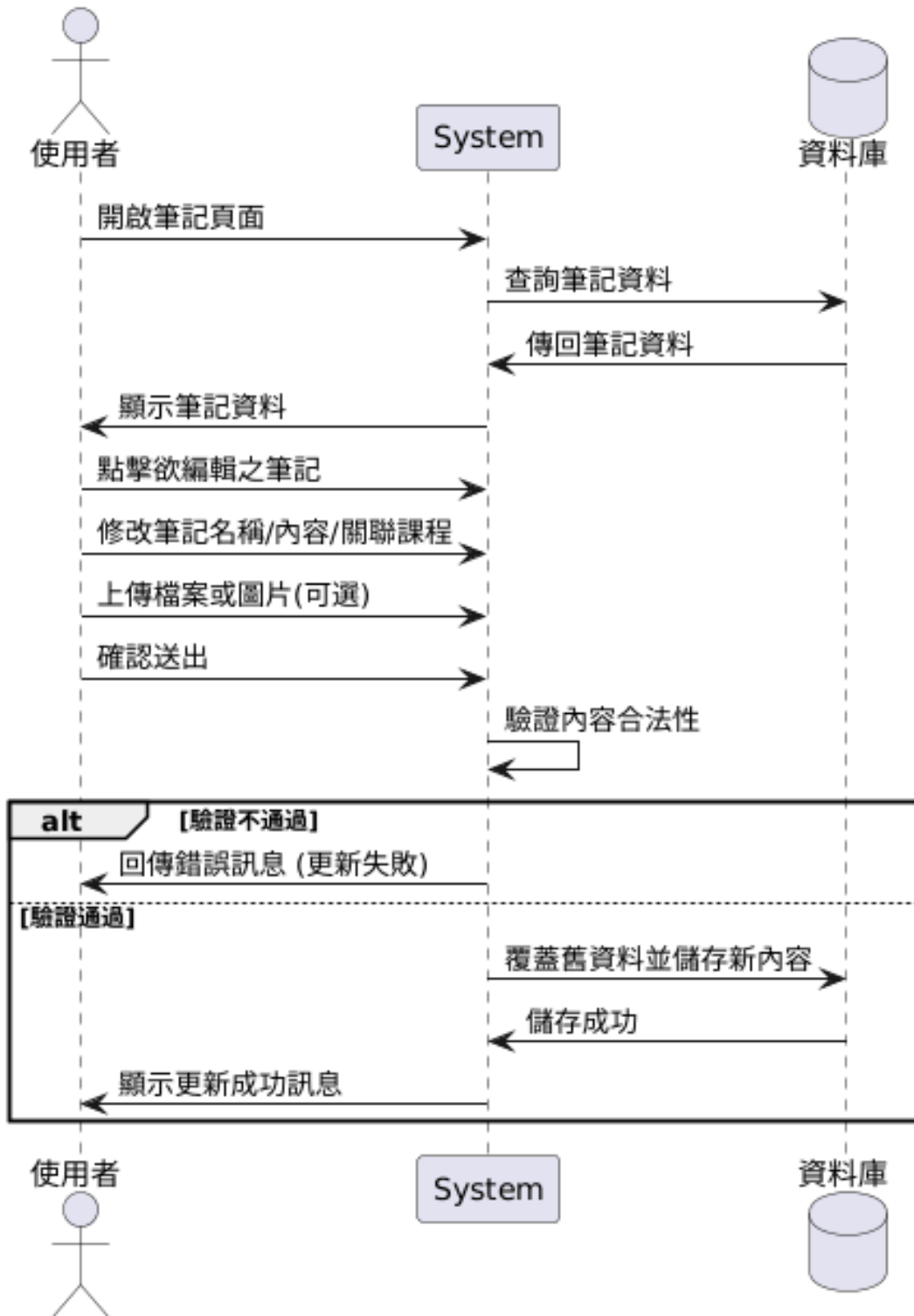
圖 6-1-11 循序圖之編輯筆記
