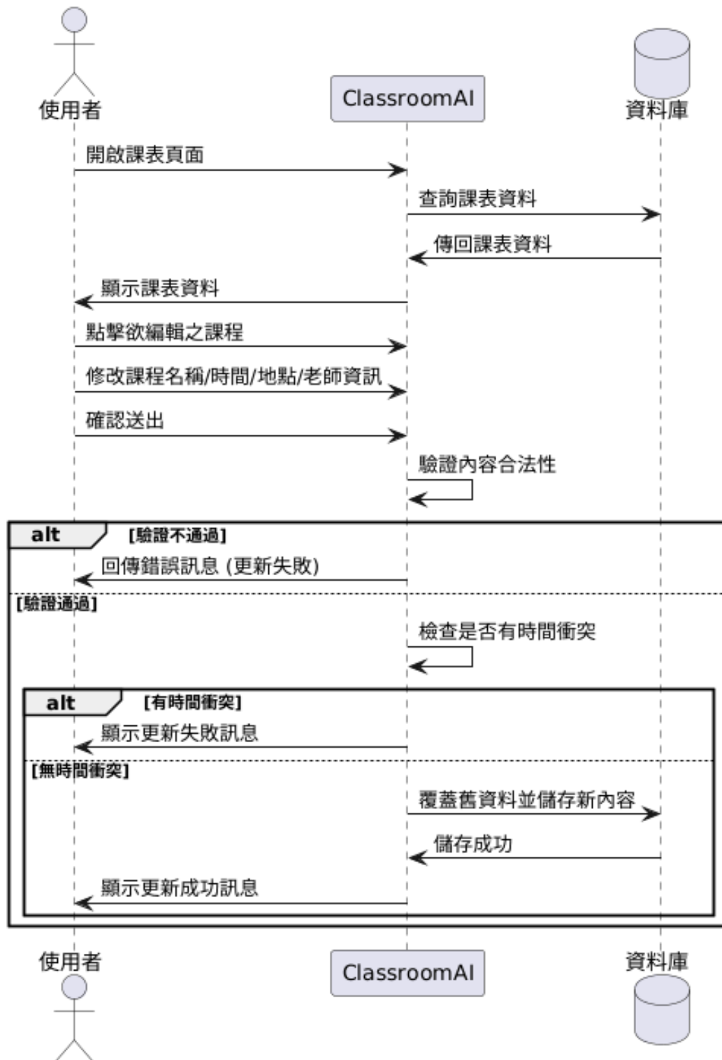
圖 6-1-3 循序圖之編輯課表
