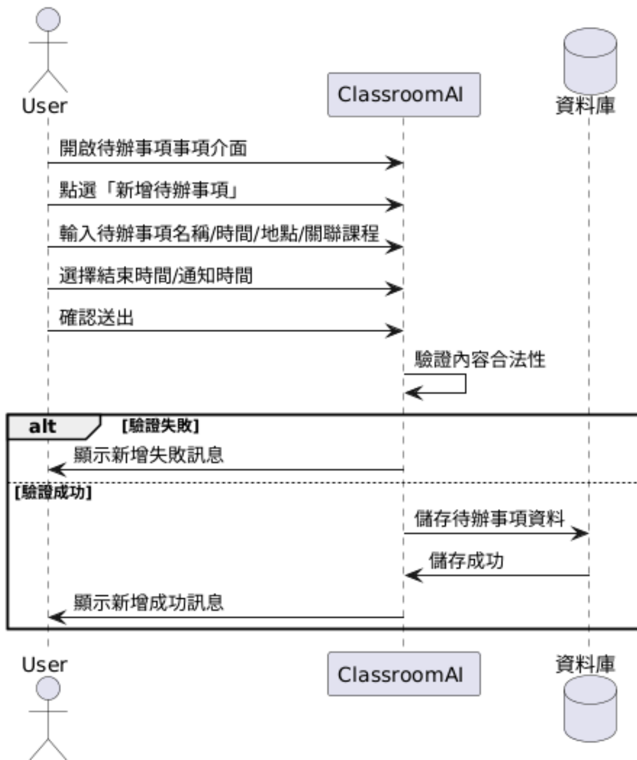
圖 6-1-6 循序圖之新增待辦事項
