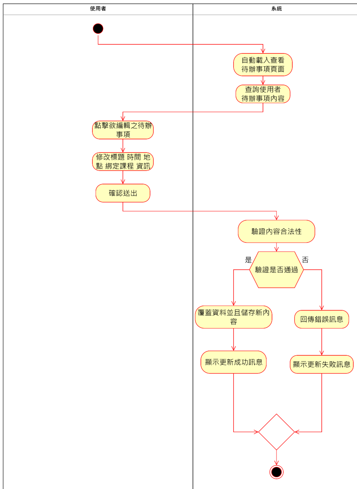
圖 5-3-7 活動圖之編輯待辦事項
