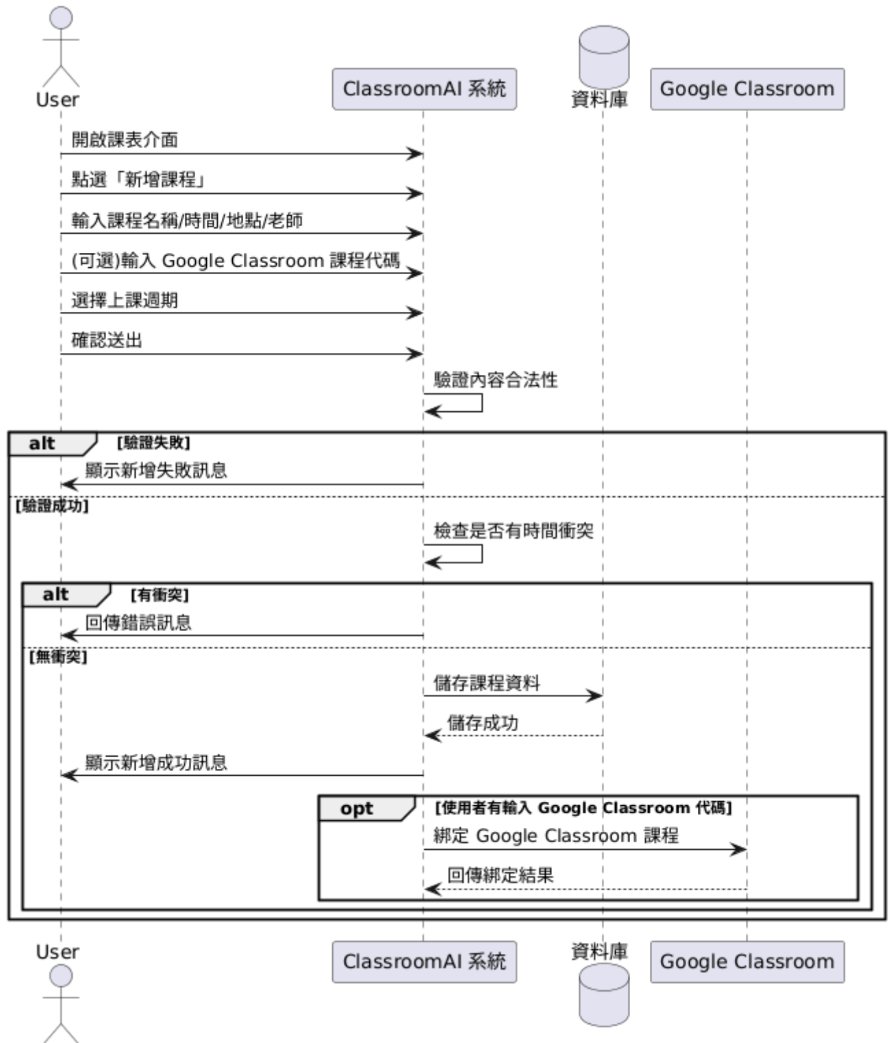
圖 6-1-2 循序圖之課表新增
