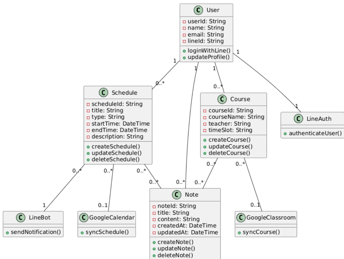
圖 5-4-1 分析類別圖
