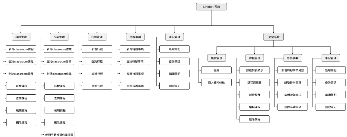
圖 3-1-2 系統架構圖
