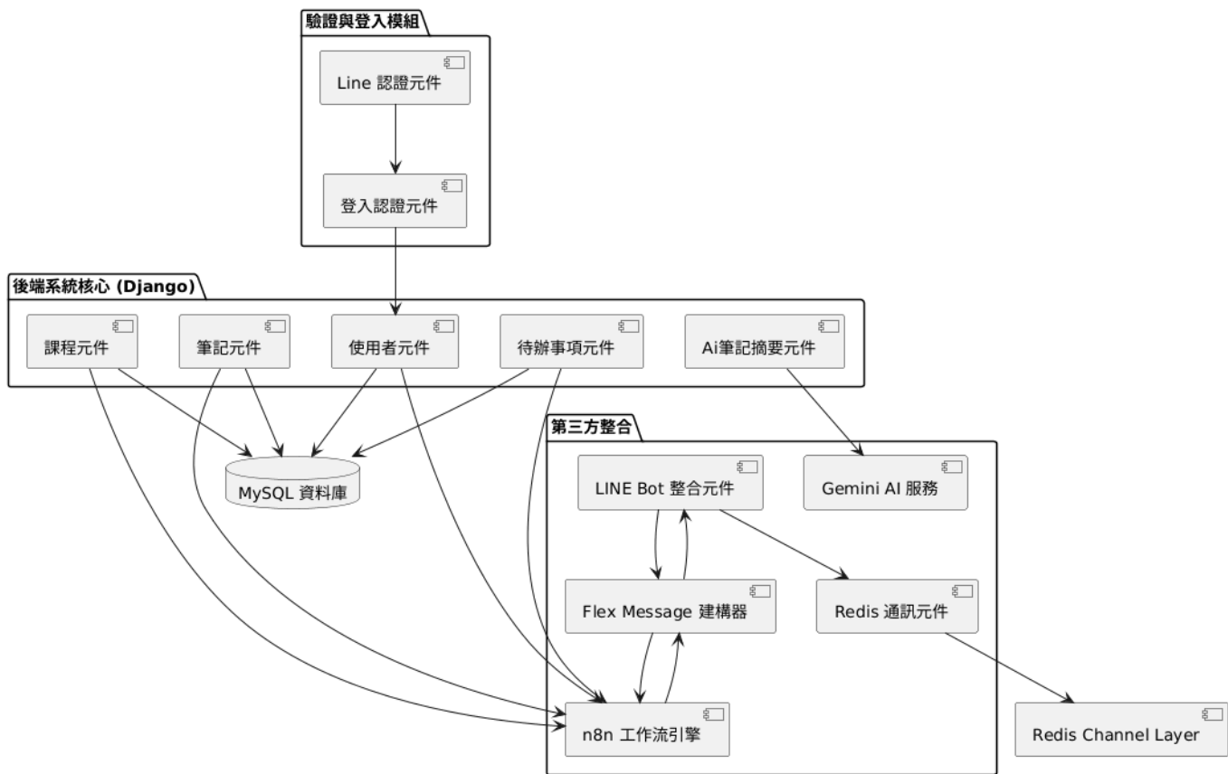
圖 7-3-1 元件圖
