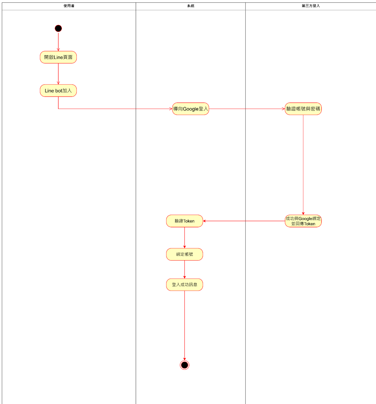
圖 5-3-1 活動圖之使用者登入
