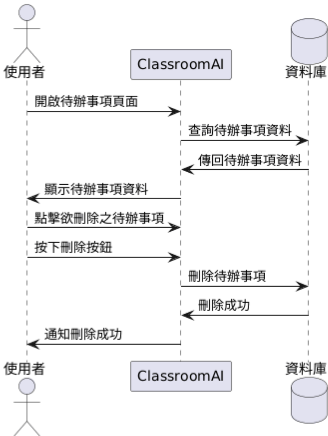
圖 6-1-8 循序圖之刪除待辦事項
