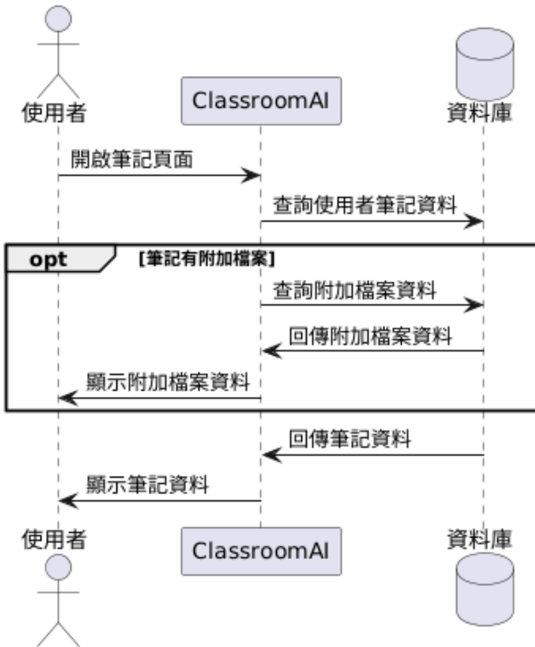
圖 6-1-13 循序圖之查看筆記
