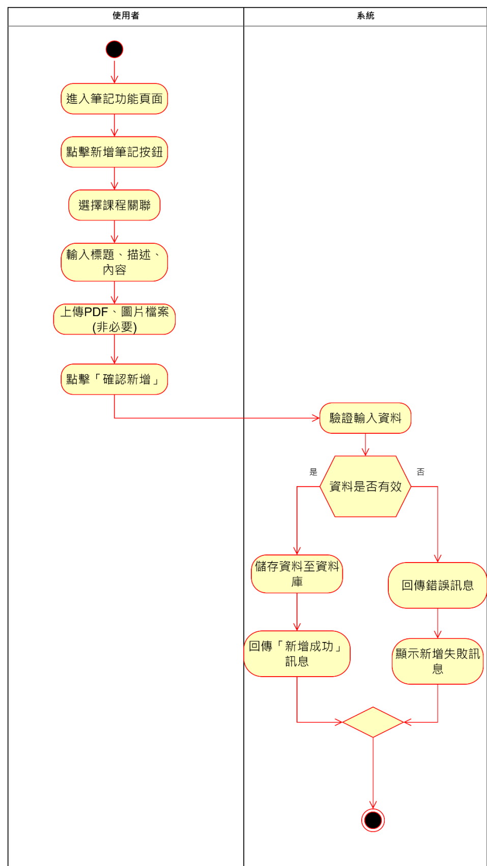
圖 5-3-10 活動圖之新增筆記
