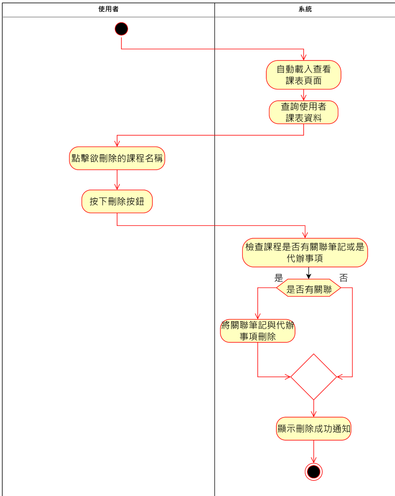
圖 5-3-4 活動圖之刪除課程
