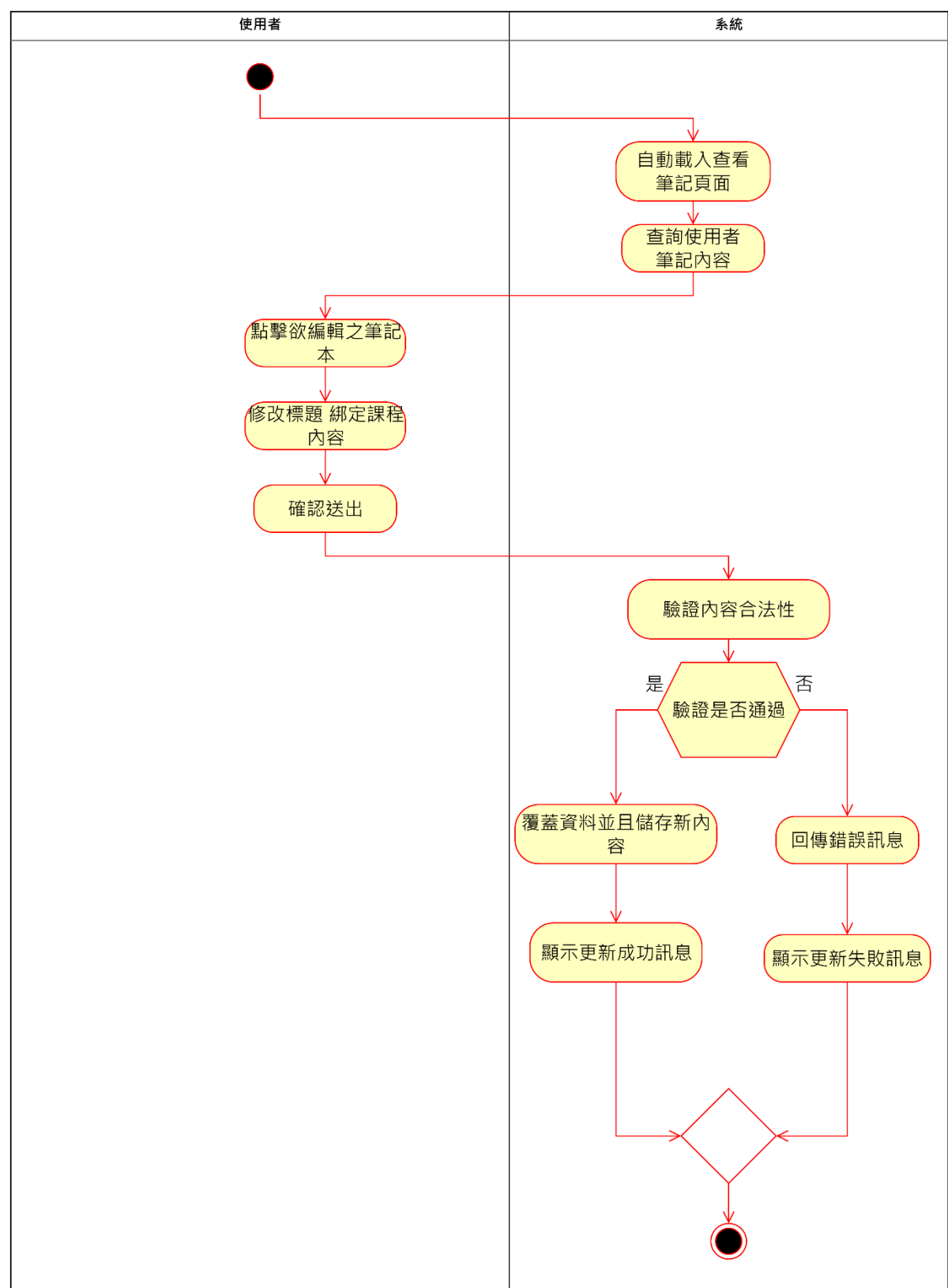
圖 5-3-11 活動圖之編輯筆記
