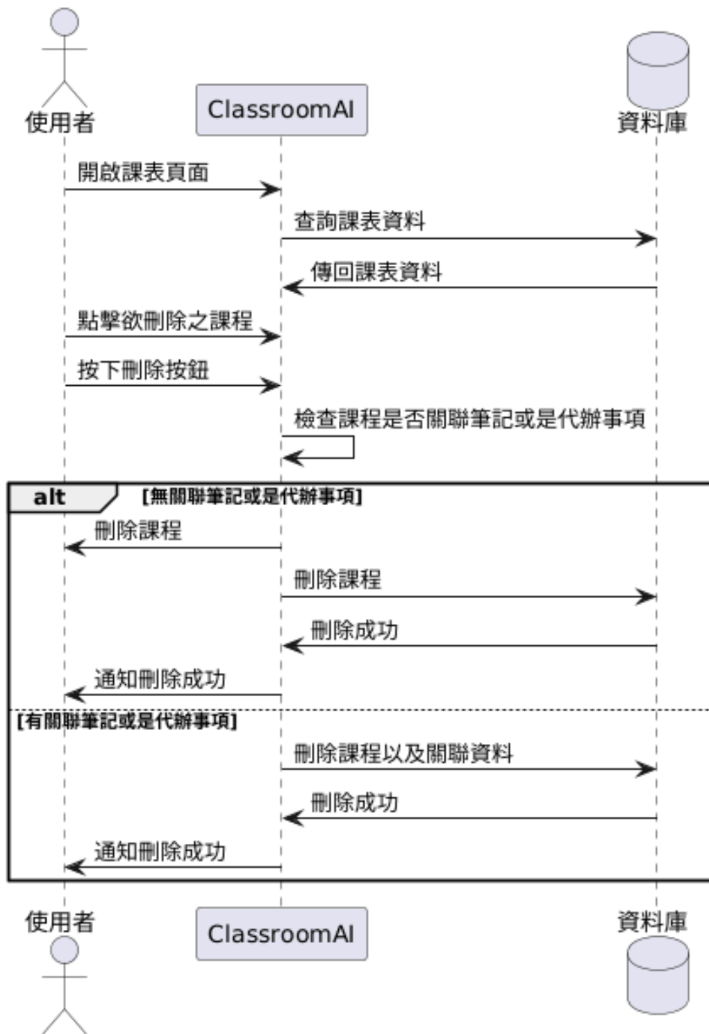
圖 6-1-4 循序圖之刪除課程
