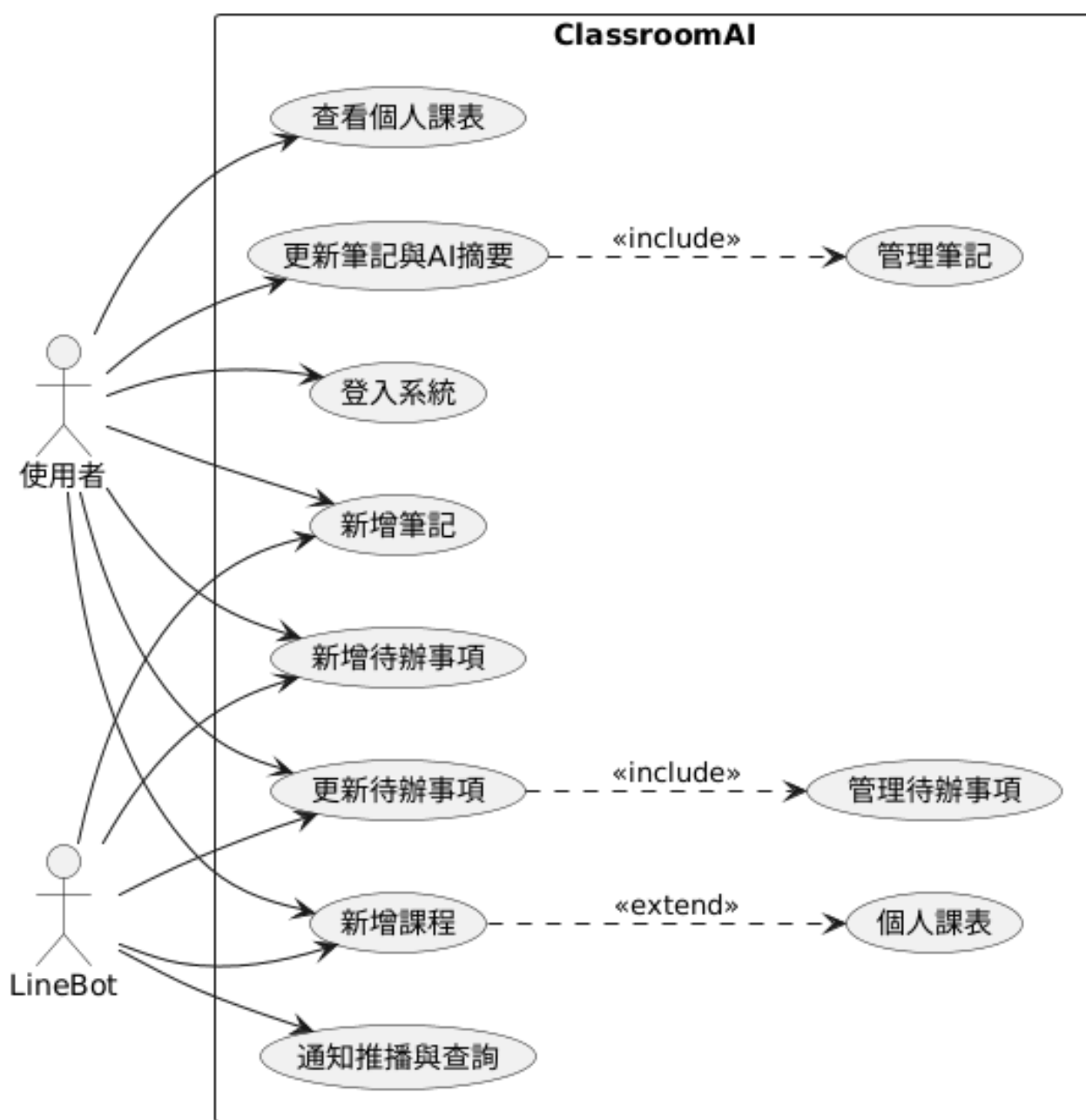
圖 5-2-1 使用個案圖
