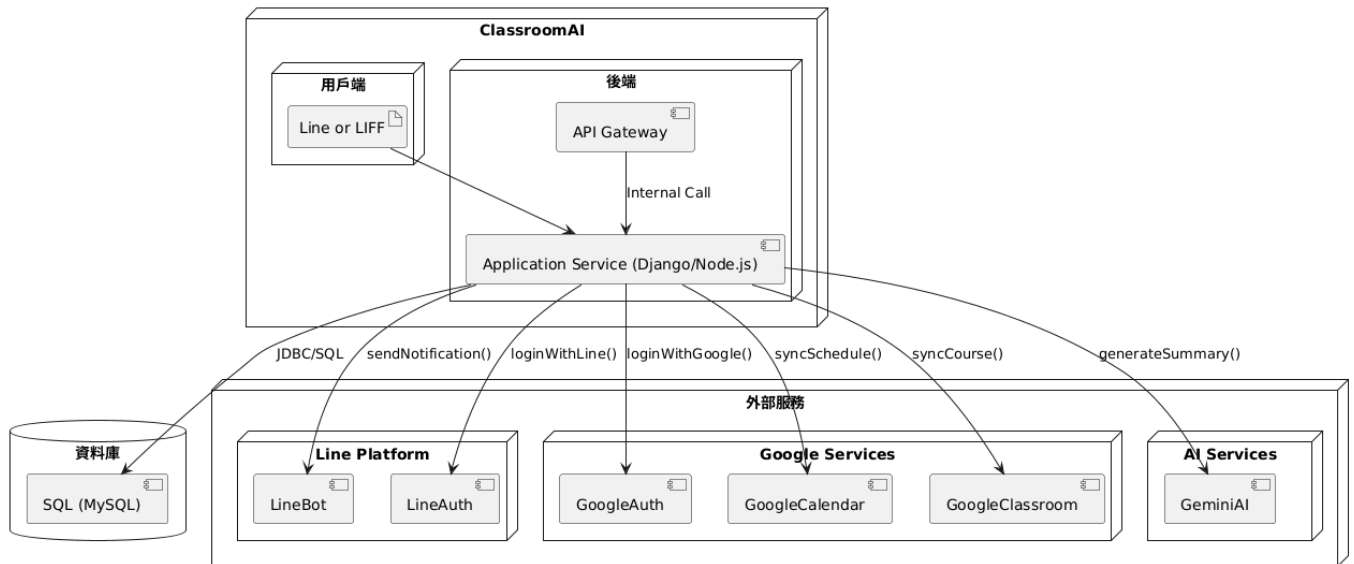
圖 7-1-1 部署圖
