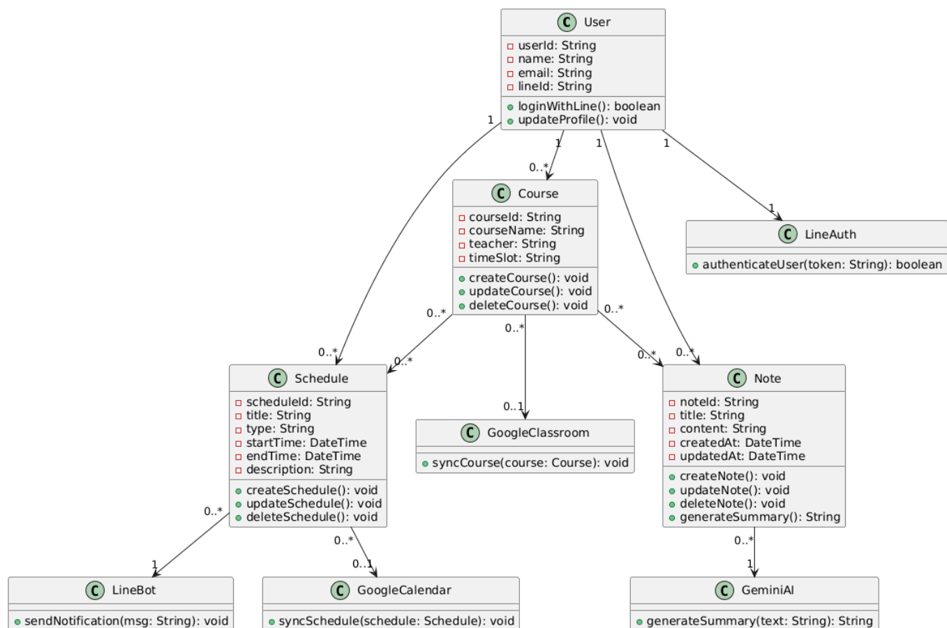
圖 6-2-1 設計類別圖
