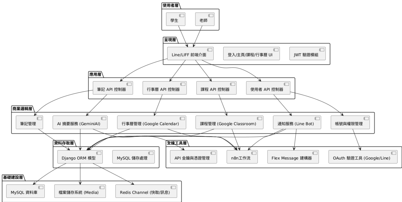
圖 7-2-1 套件圖
