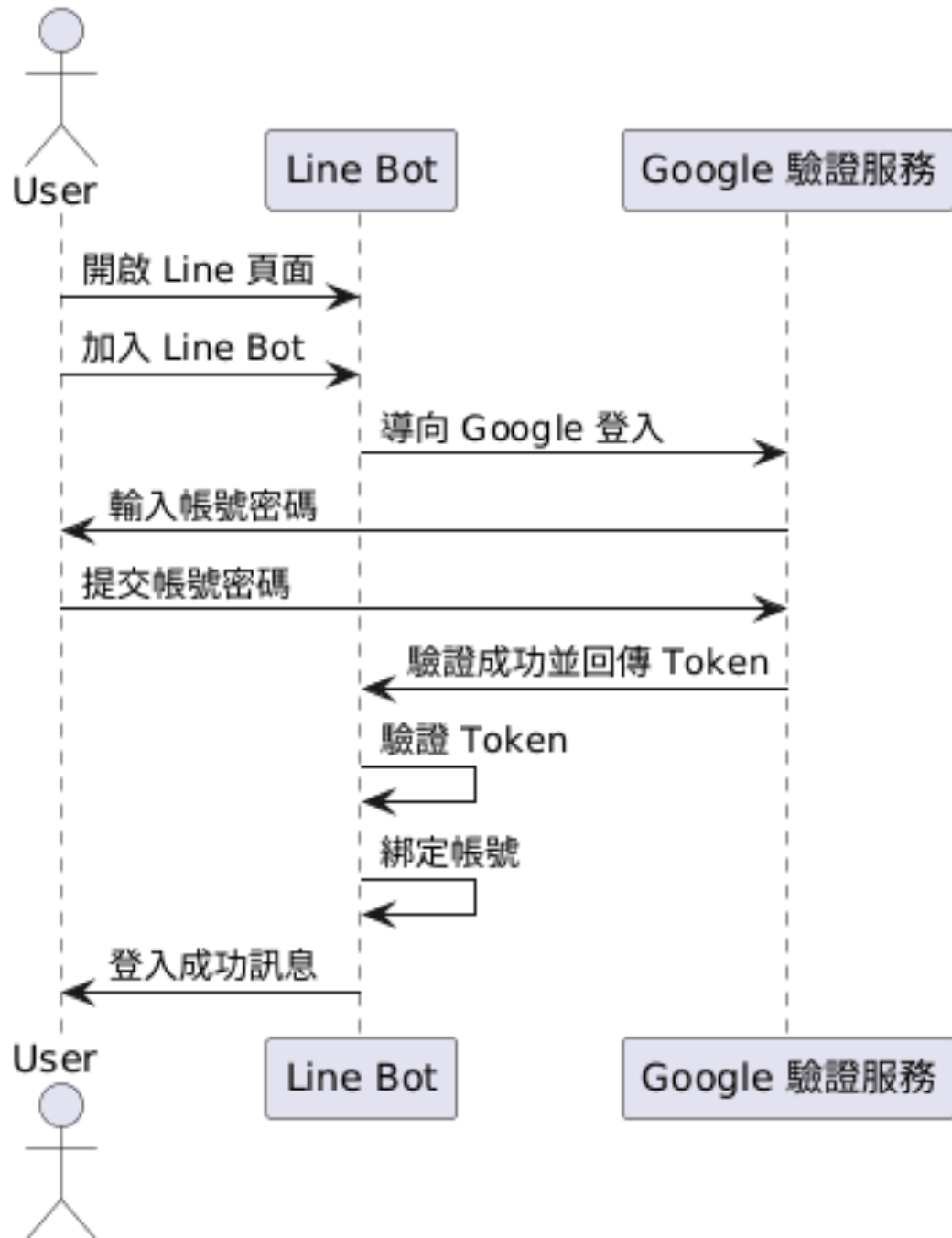
圖 6-1-1 循序圖之使用者登入
