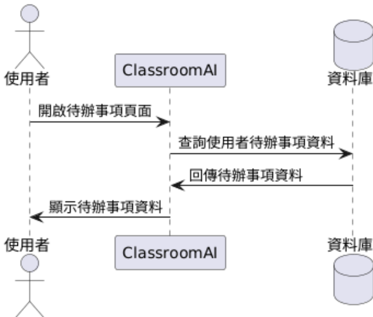
圖 6-1-9 循序圖之查看待辦事項
