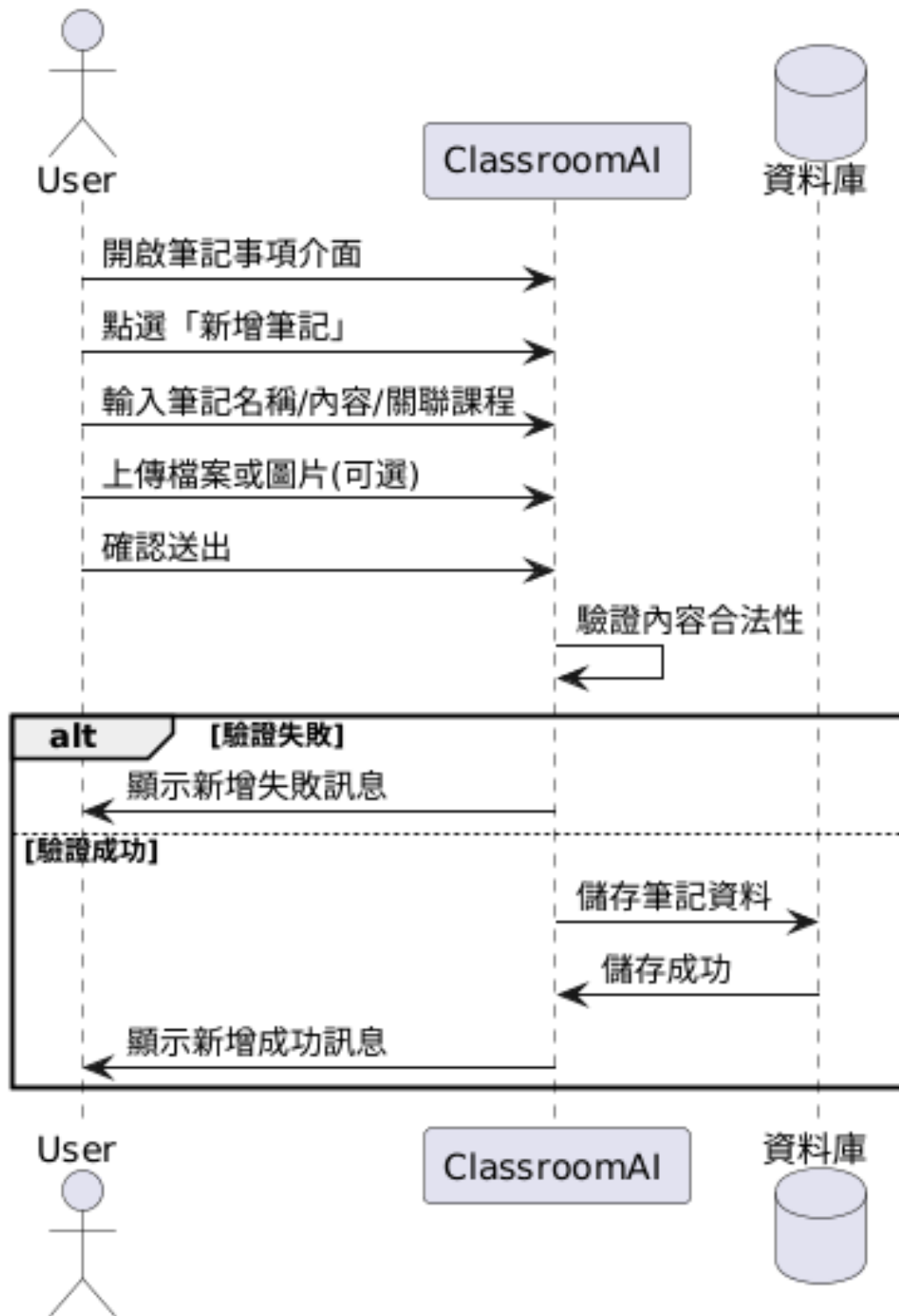
圖 6-1-10 循序圖之新增筆記
