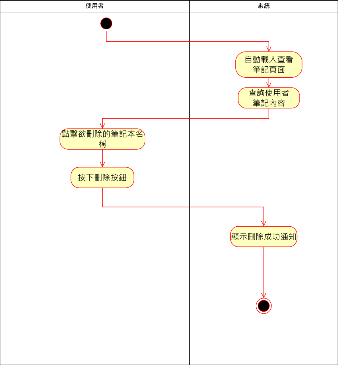
圖 5-3-12 活動圖之刪除筆記
