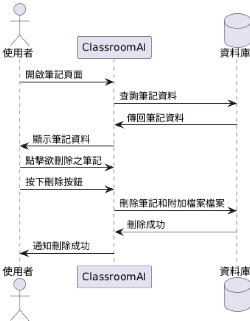
圖 6-1-12 循序圖之刪除筆記
