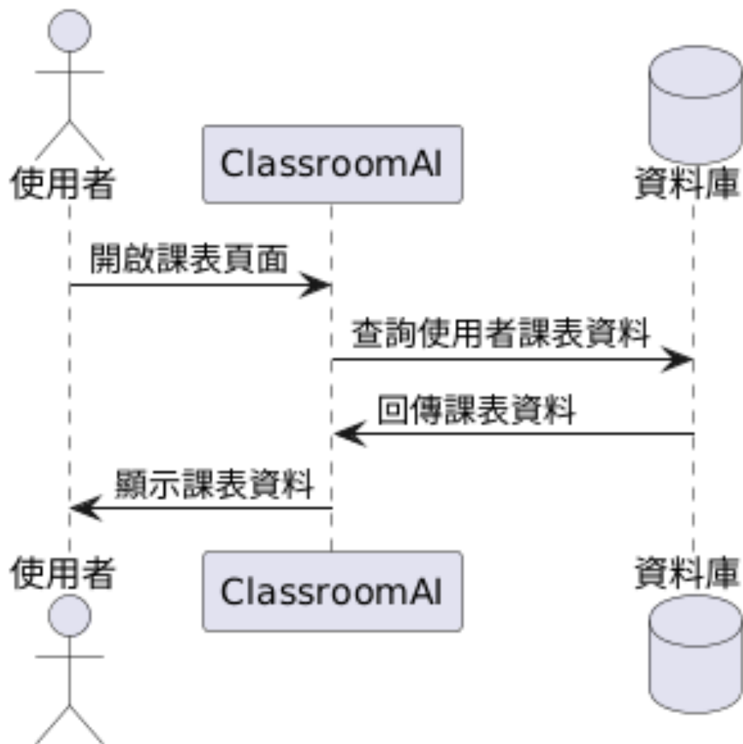
圖 6-1-5 循序圖之查看課程
