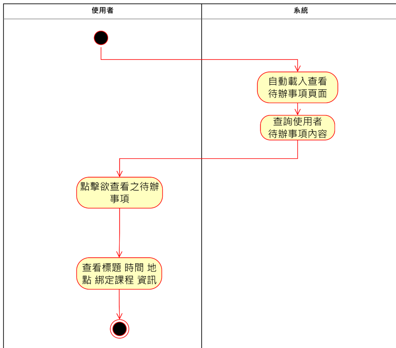
圖 5-3-9 活動圖之查看待辦事項
