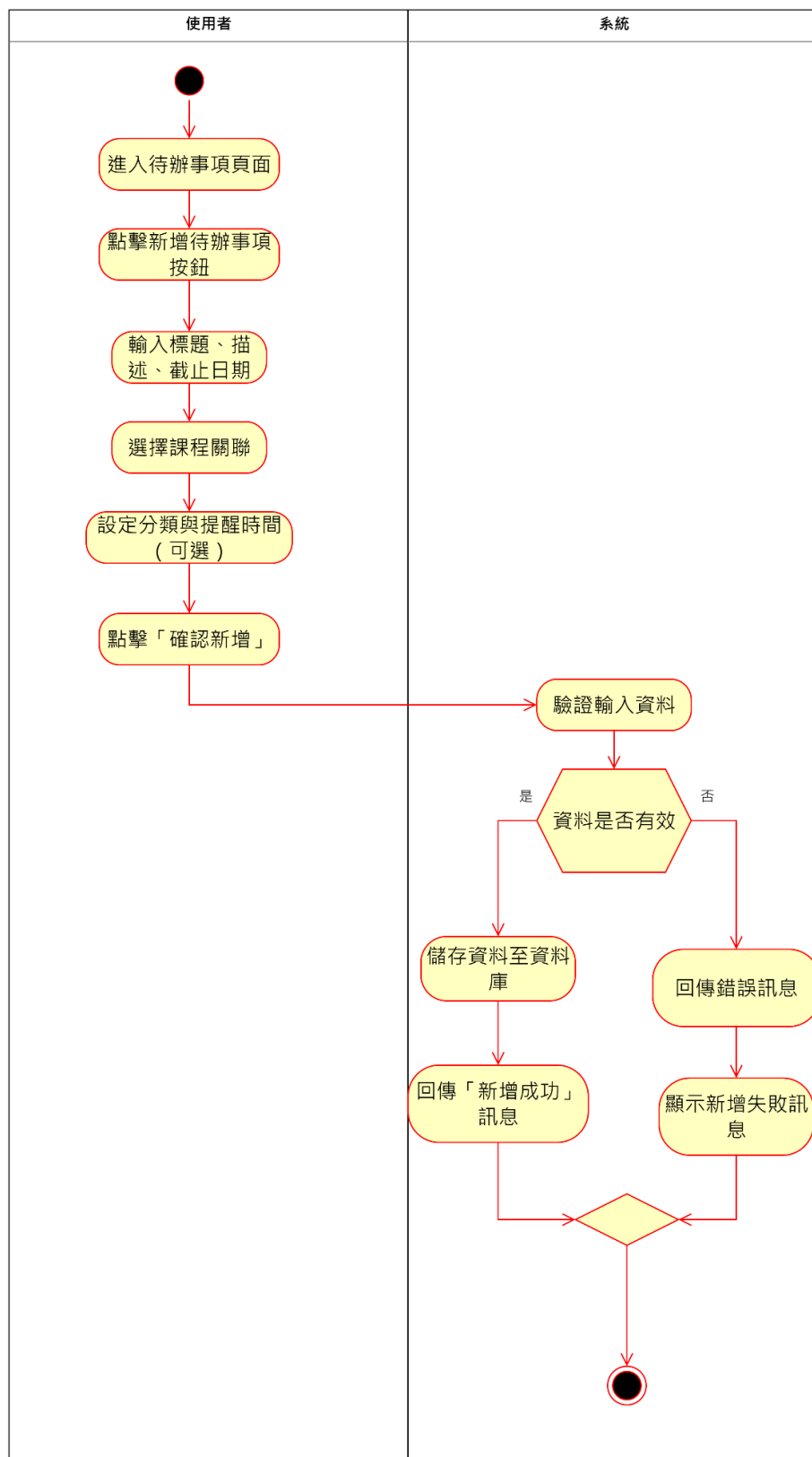
圖 5-3-6 活動圖之新增待辦事項
