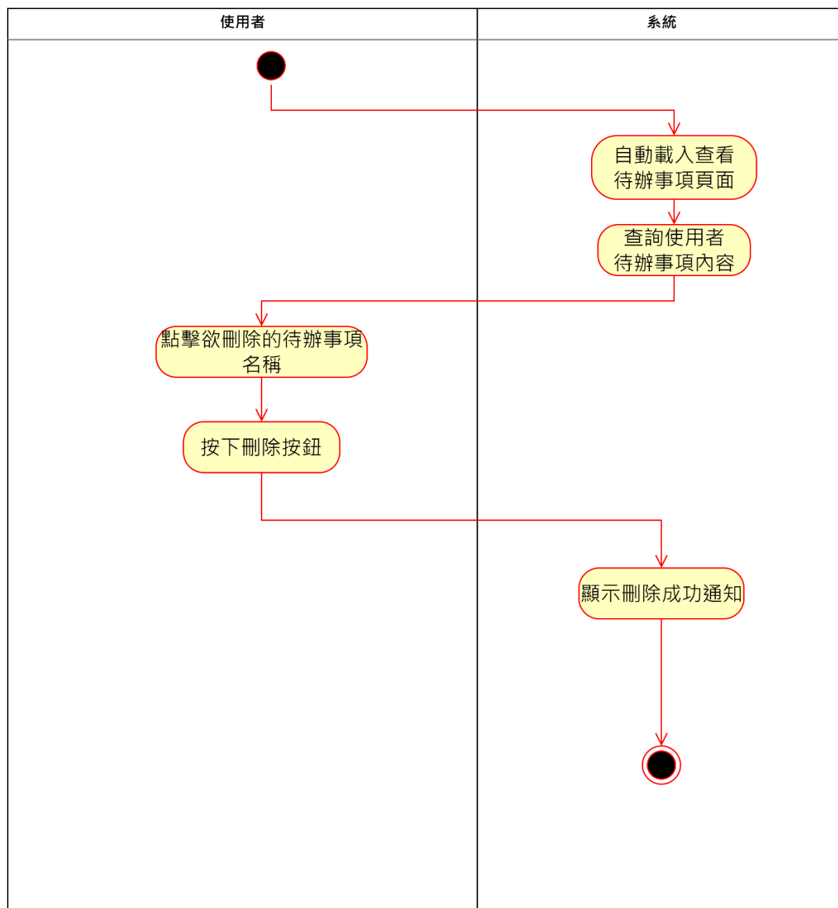
圖 5-3-8 活動圖之刪除待辦事項
