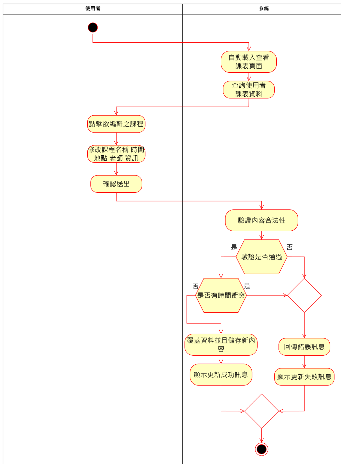
圖 5-3-3 活動圖之編輯課程
